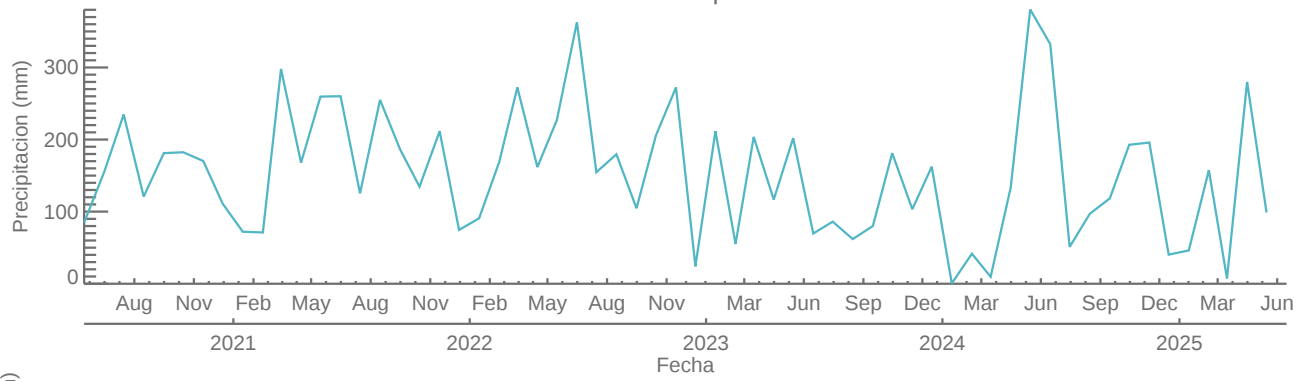
434 – Museo de Antioquia – Pluviometro
