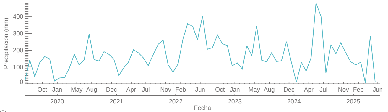
383 – Salinas Caldas – Pluviometro
