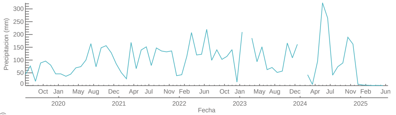
378 – Edificio Camacol – Pluviometro
