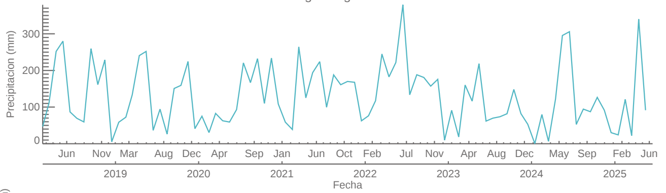
281 – Megacolegio – Pluviometro
