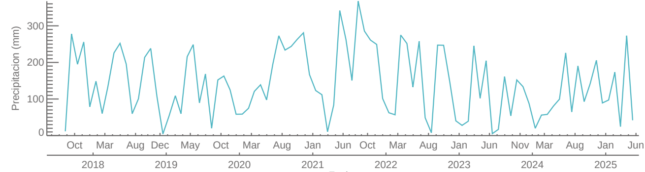
227 – Sonson – Pluviometro
