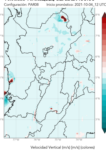
Pronóstico SIATA: Velocidad Vertical (m/s) 500 hPa 2021-10-05 07:00:00
