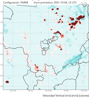
Pronóstico SIATA: Velocidad Vertical (m/s) 500 hPa 2021-10-05 04:00:00
