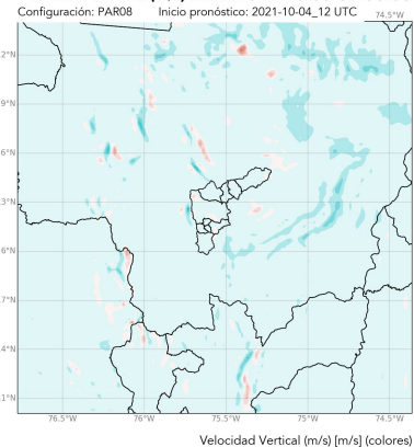
Pronóstico SIATA: Velocidad Vertical (m/s) 500 hPa 2021-10-05 07:00:00
