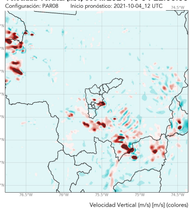
Pronóstico SIATA: Velocidad Vertical (m/s) 500 hPa 2021-10-04 22:00:00
