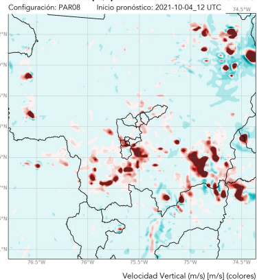
Pronóstico SIATA: Velocidad Vertical (m/s) 500 hPa 2021-10-05 01:00:00
