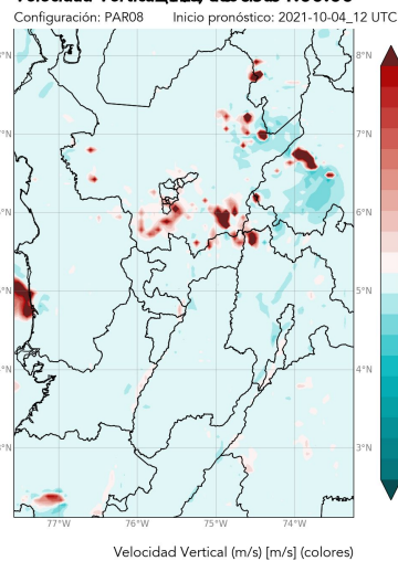
Pronóstico SIATA: Velocidad Vertical (m/s) 500 hPa 2021-10-05 01:00:00
