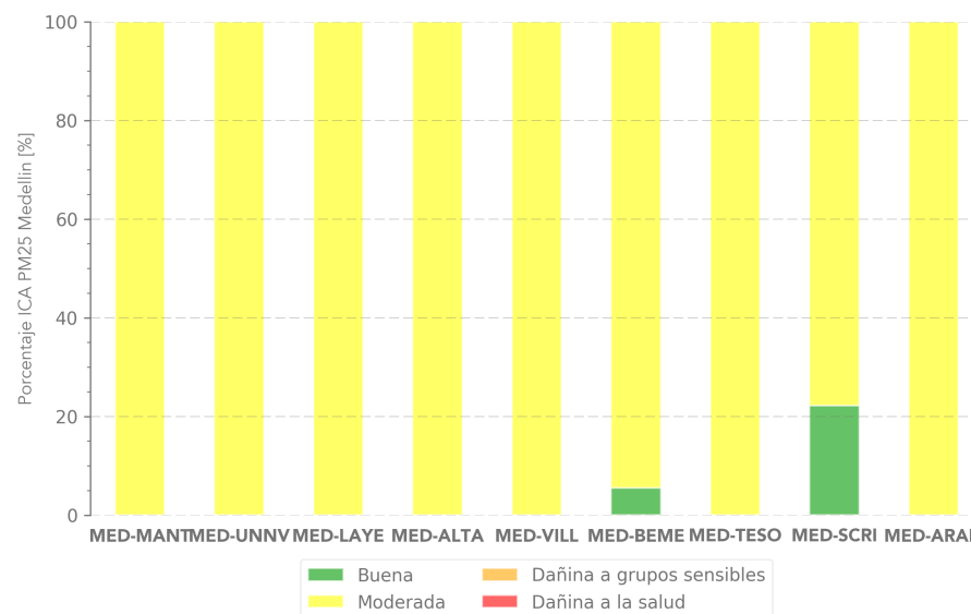
Porcentaje ICA PM2.5
