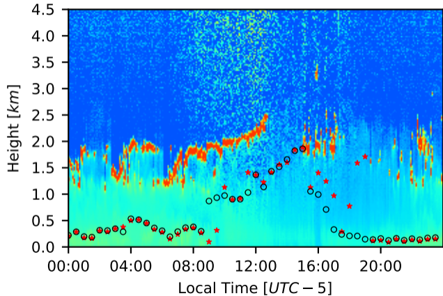
03-04-2014 SIATA Ceilometer Retrievals
