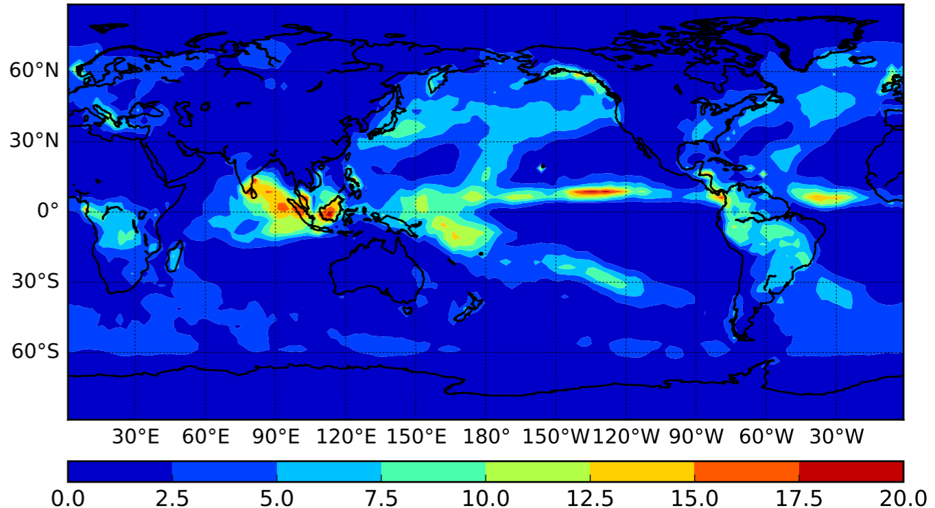
GPCP Precipitación Precipitación (mm/día) 1979/11
