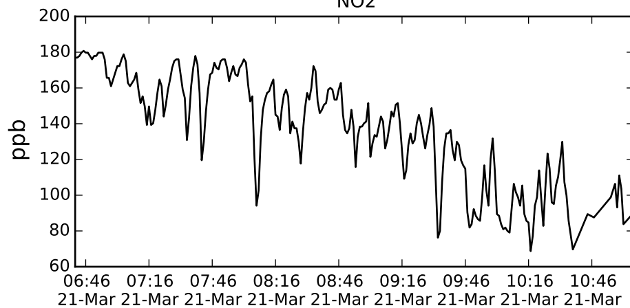
NO2
