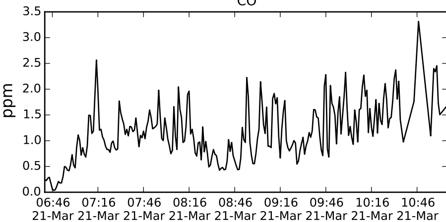
CO
