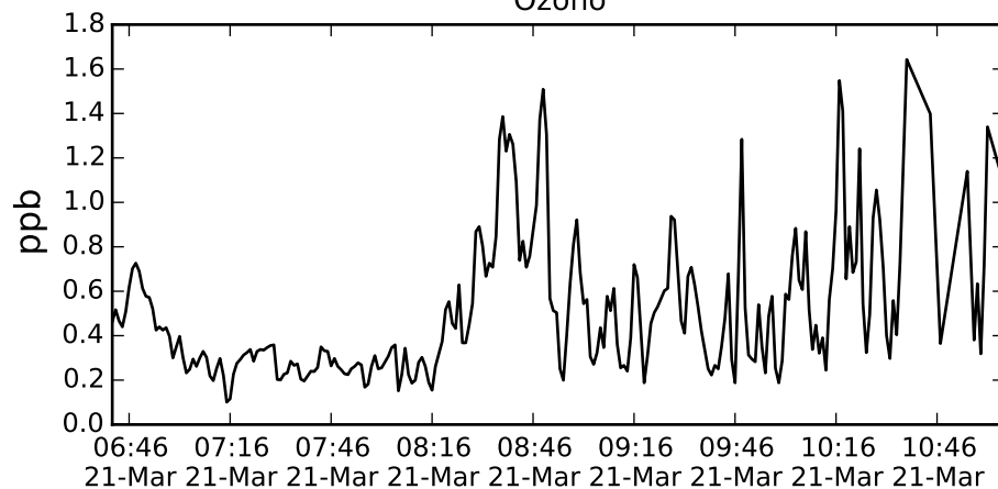
Ozono
