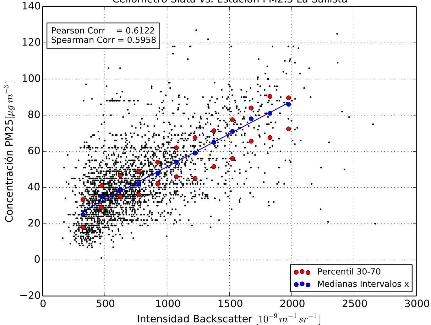
Ceilómetro Siata vs. Estación PM2.5 La Sallista
