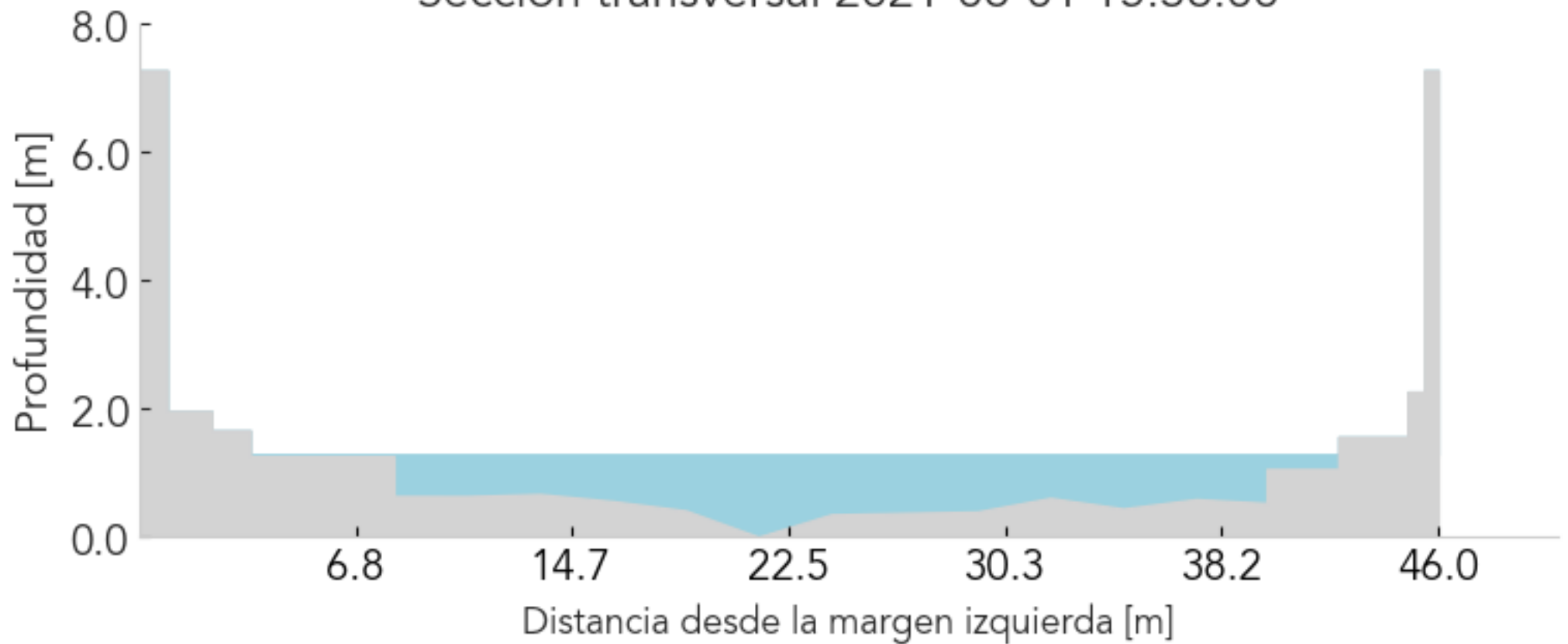
Sección transversal 2021-06-01 15:38:00
