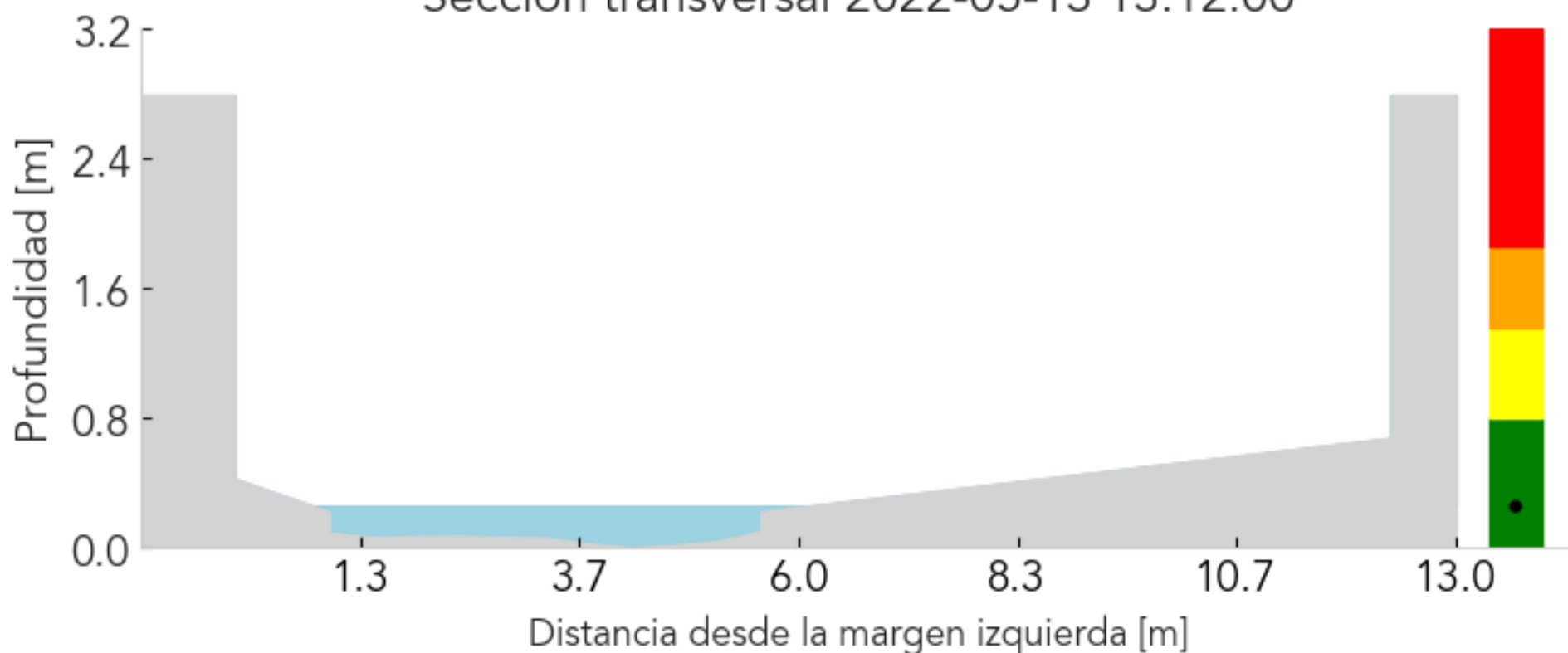
Sección transversal 2022-05-13 13:12:00
