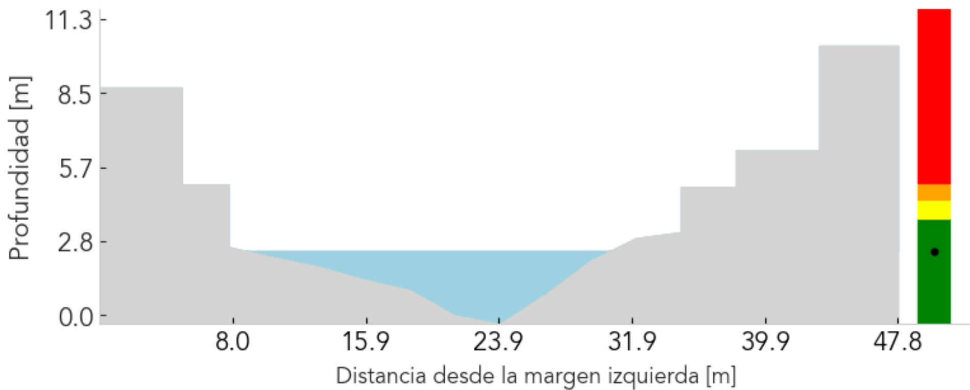
Sección transversal 2022-05-13 13:12:00
