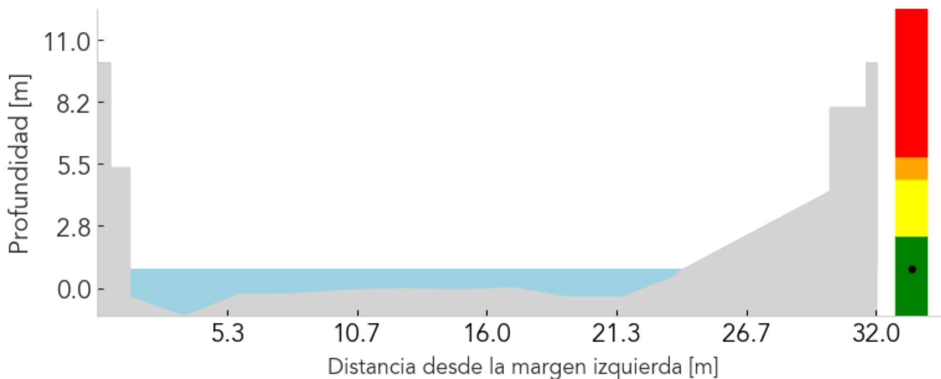
Sección transversal 2022-05-13 13:06:00
