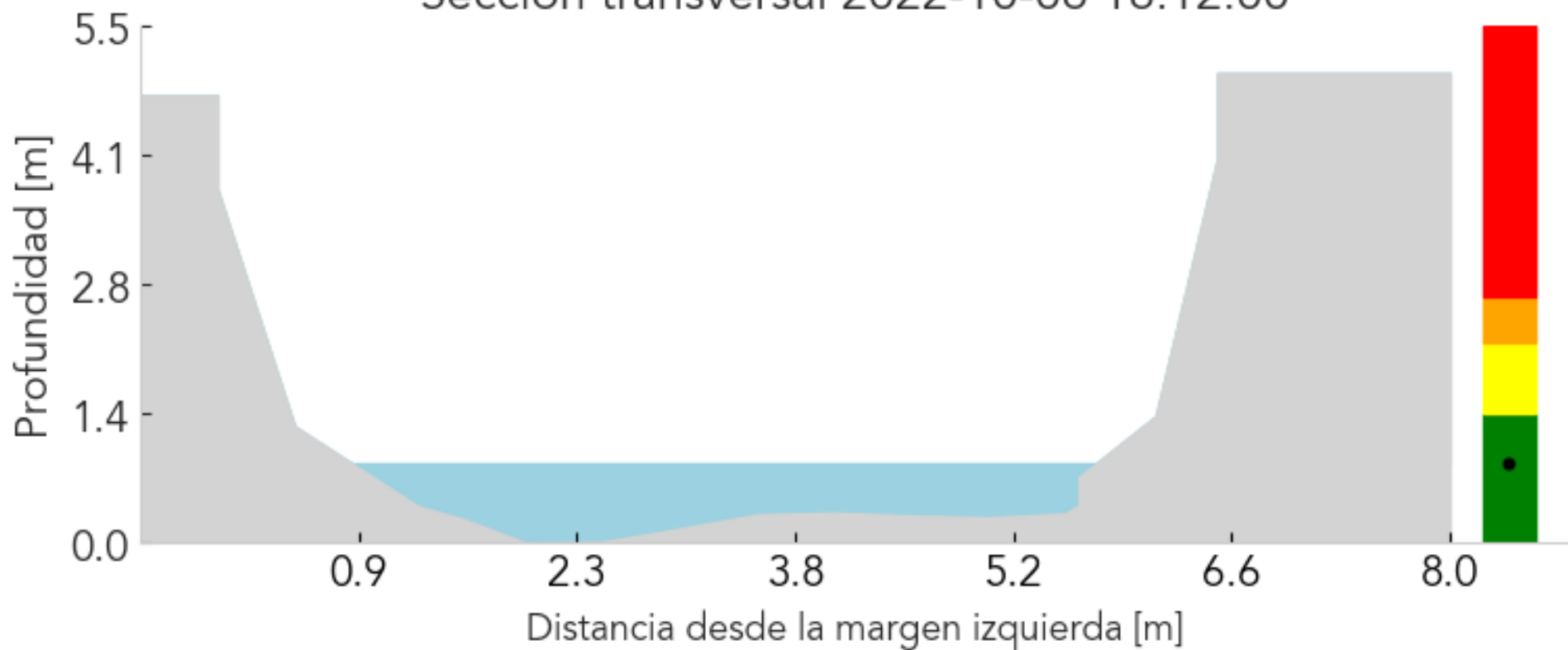
Sección transversal 2022-10-06 18:12:00
