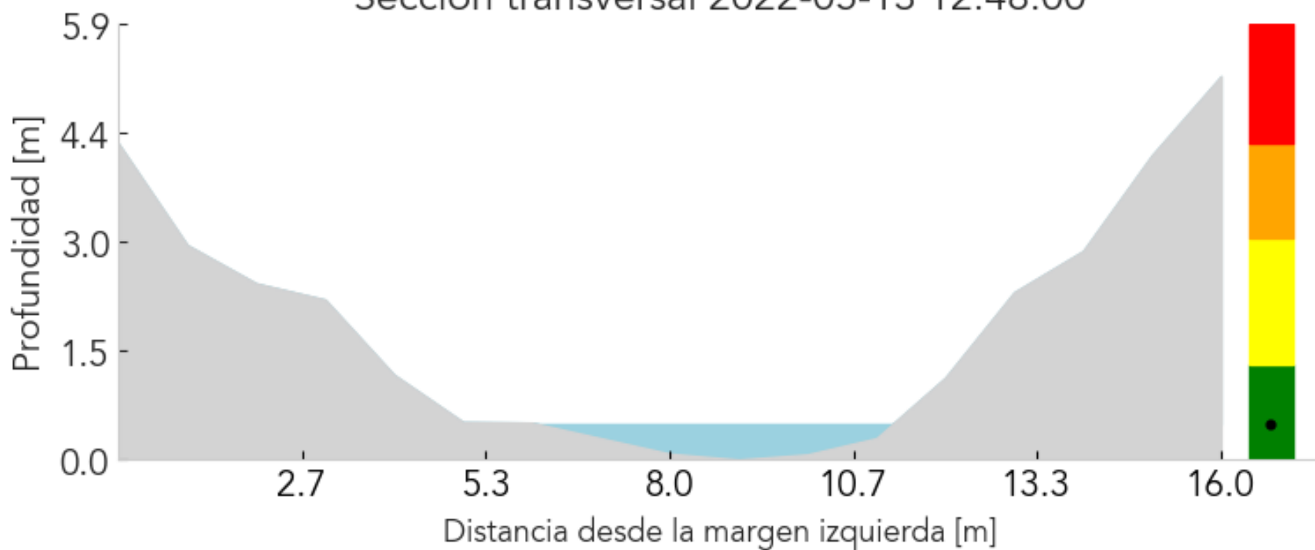
Sección transversal 2022-05-13 12:48:00
