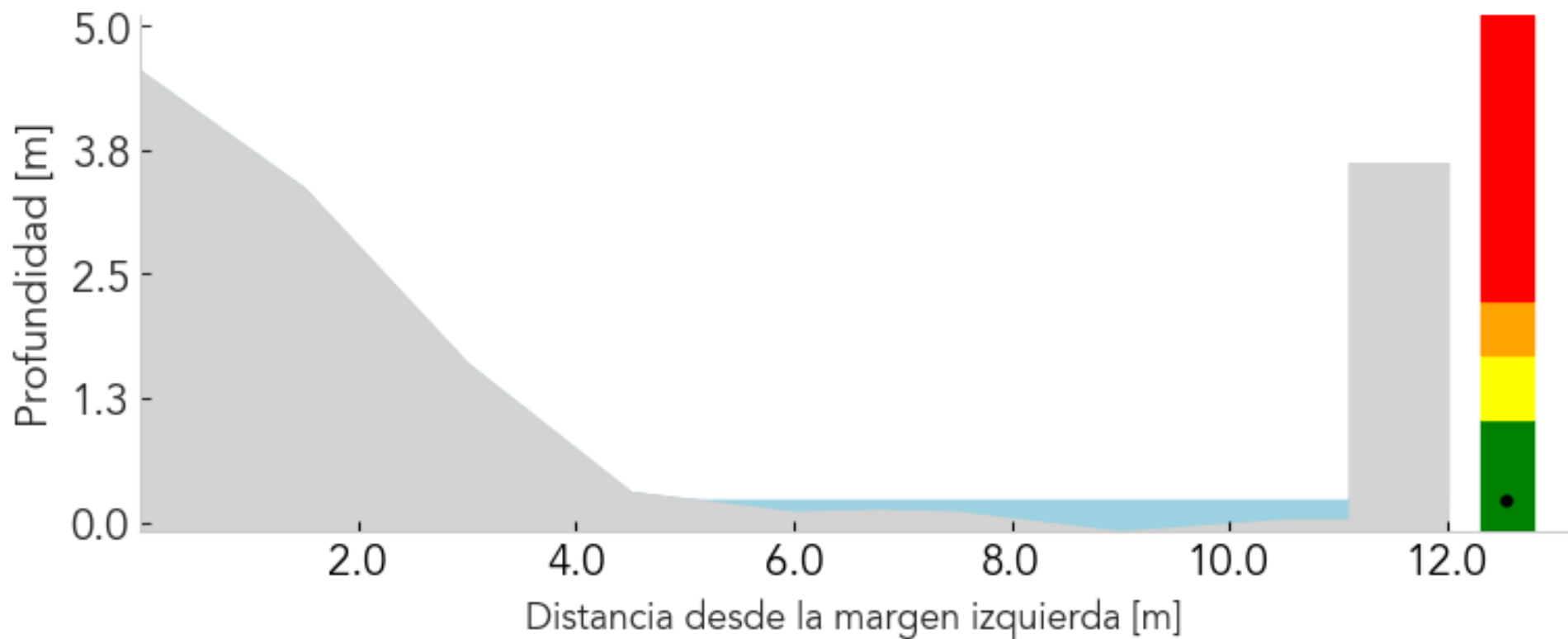
Sección transversal 2022-05-13 12:48:00
