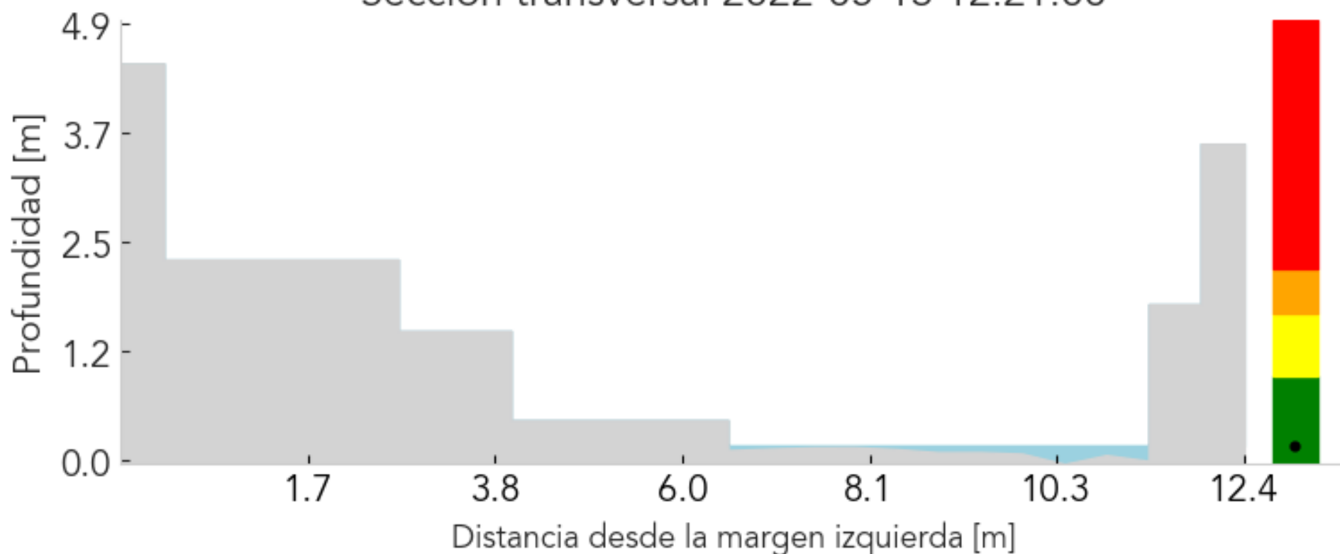
Sección transversal 2022-05-13 12:21:00
