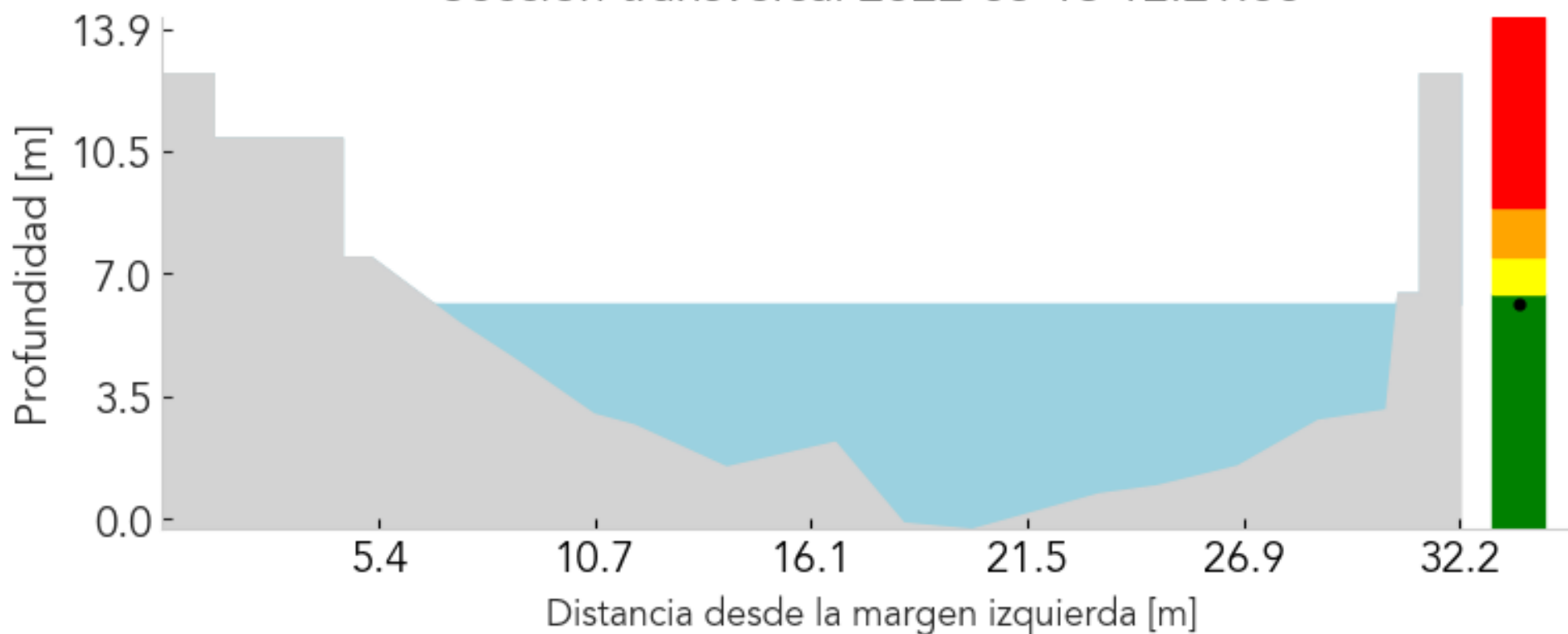
Sección transversal 2022-05-13 12:21:00
