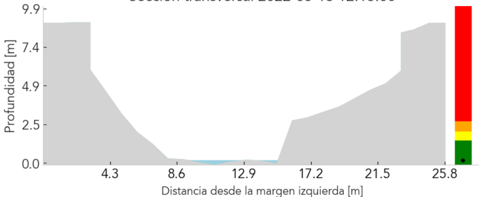
Sección transversal 2022-05-13 12:15:00
