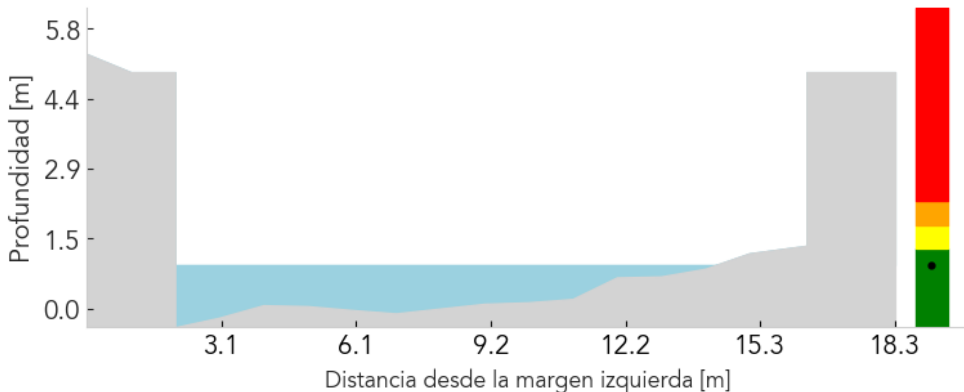
Sección transversal 2022-05-13 12:06:00
