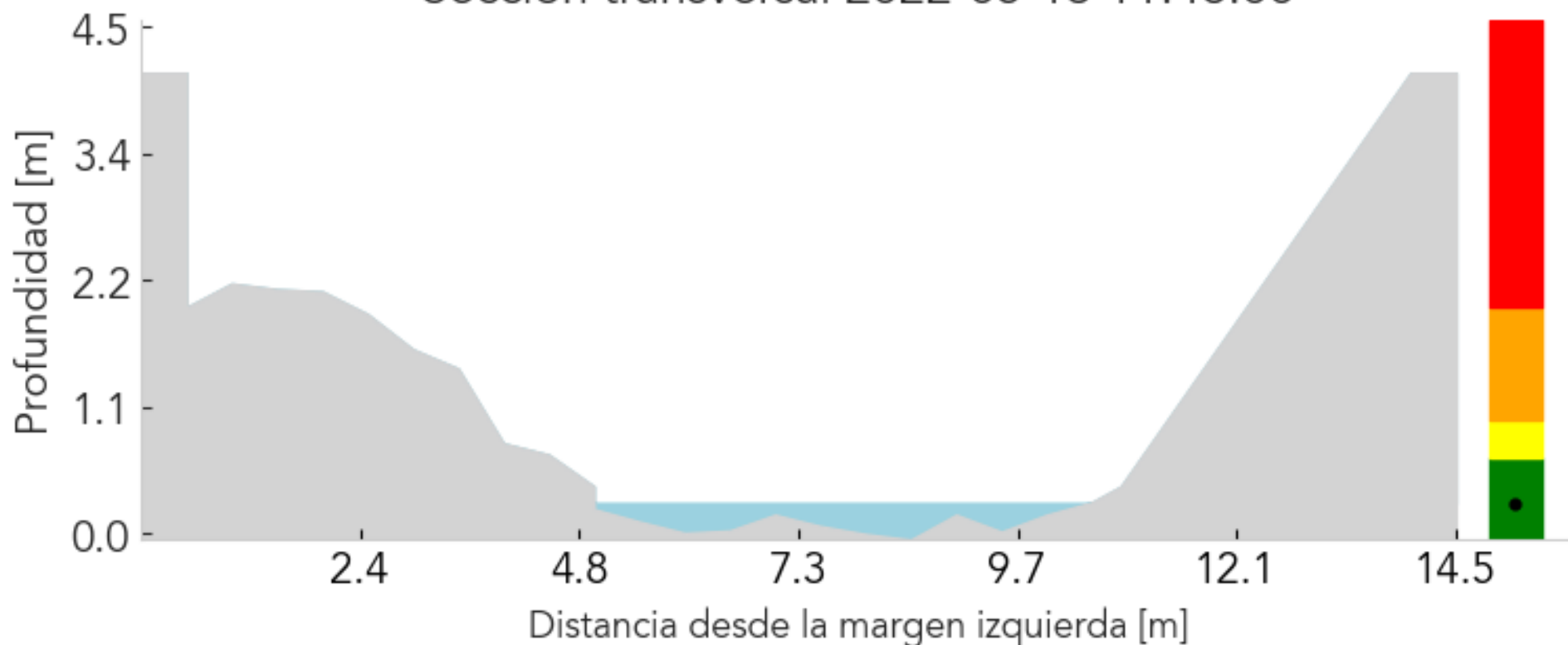
Sección transversal 2022-05-13 11:48:00
