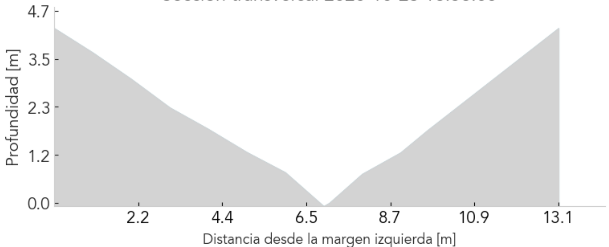
Sección transversal 2020-10-23 16:56:00
