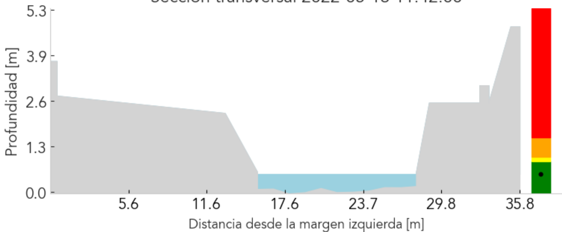
Sección transversal 2022-05-13 11:42:00
