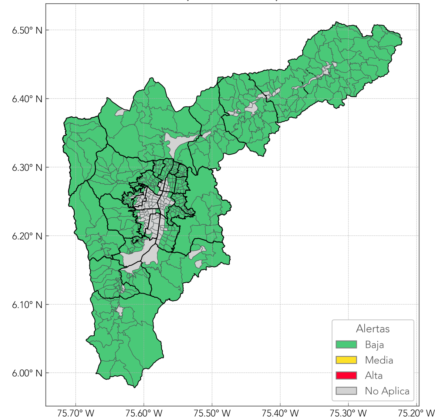
Probabilidad de ocurrencia de Movimientos en Masa (2025-12-29)
