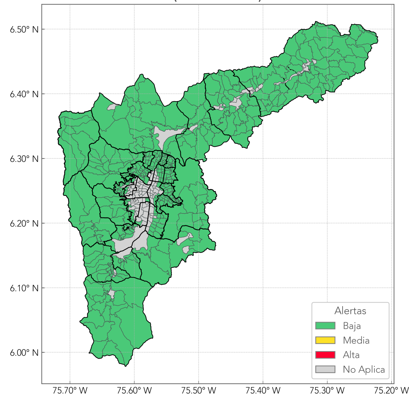
Probabilidad de ocurrencia de Movimientos en Masa (2025-11-03)
