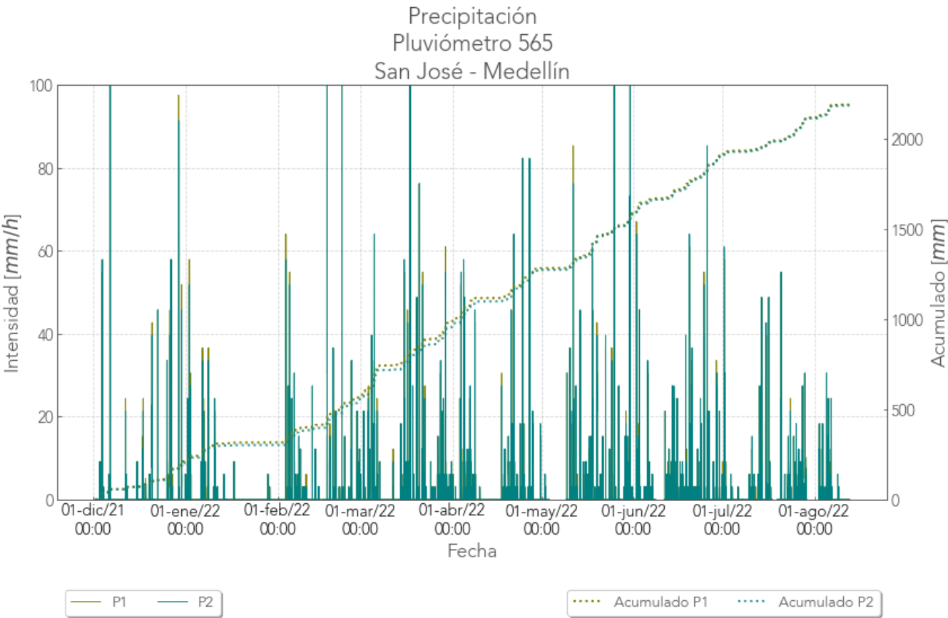
Figura 3. Histórico pluviómetro 565. Tanque vereda San José.
