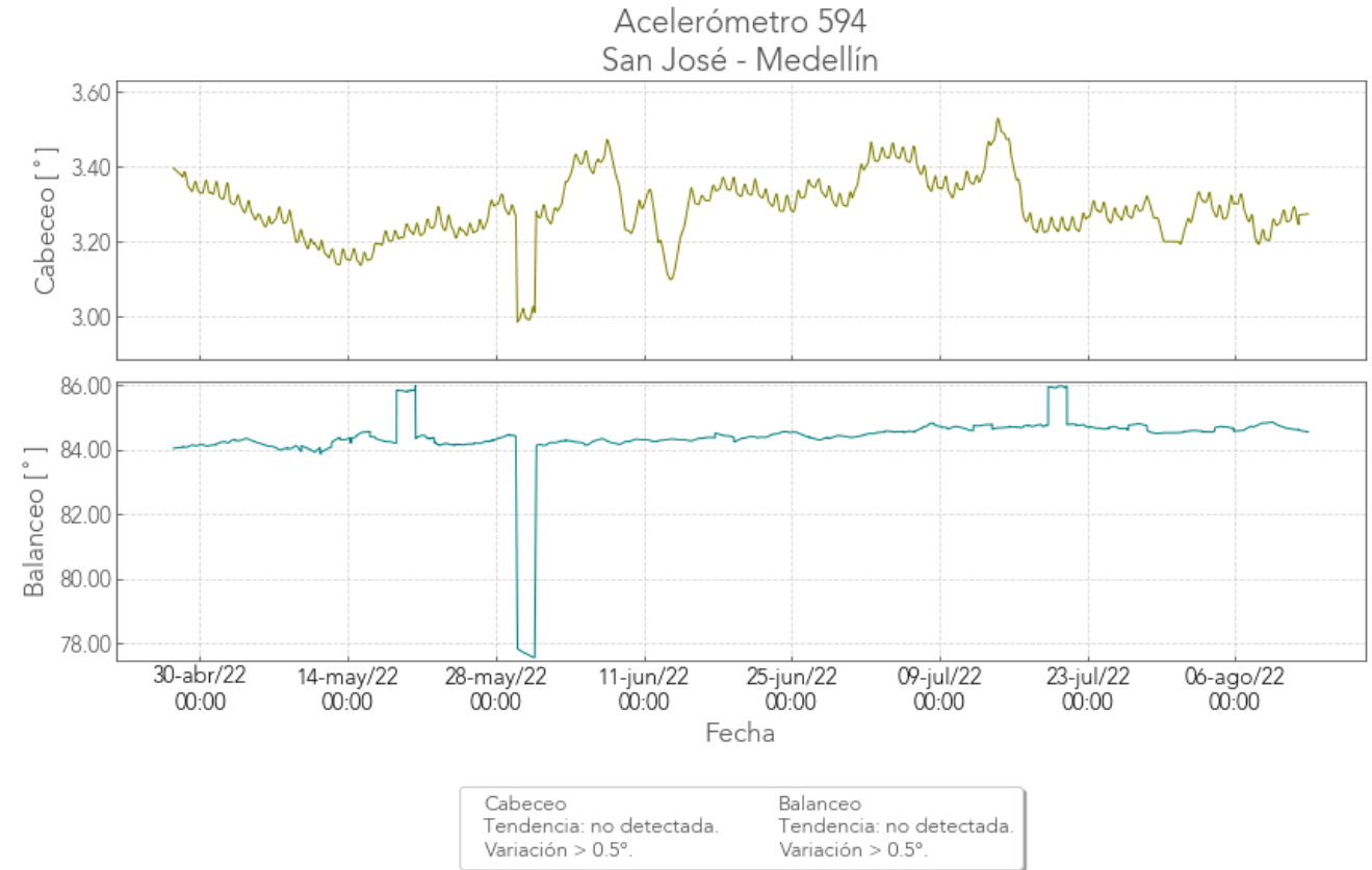
Figura 7. Histórico acelerómetro 594. Tanque vereda San José.
