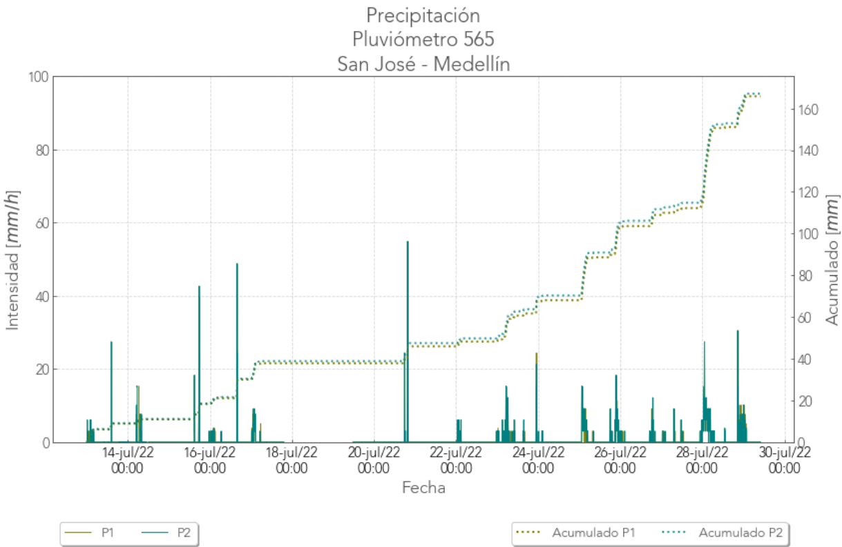
Figura 2. Registro pluviómetro 565 San José-Medellín.
