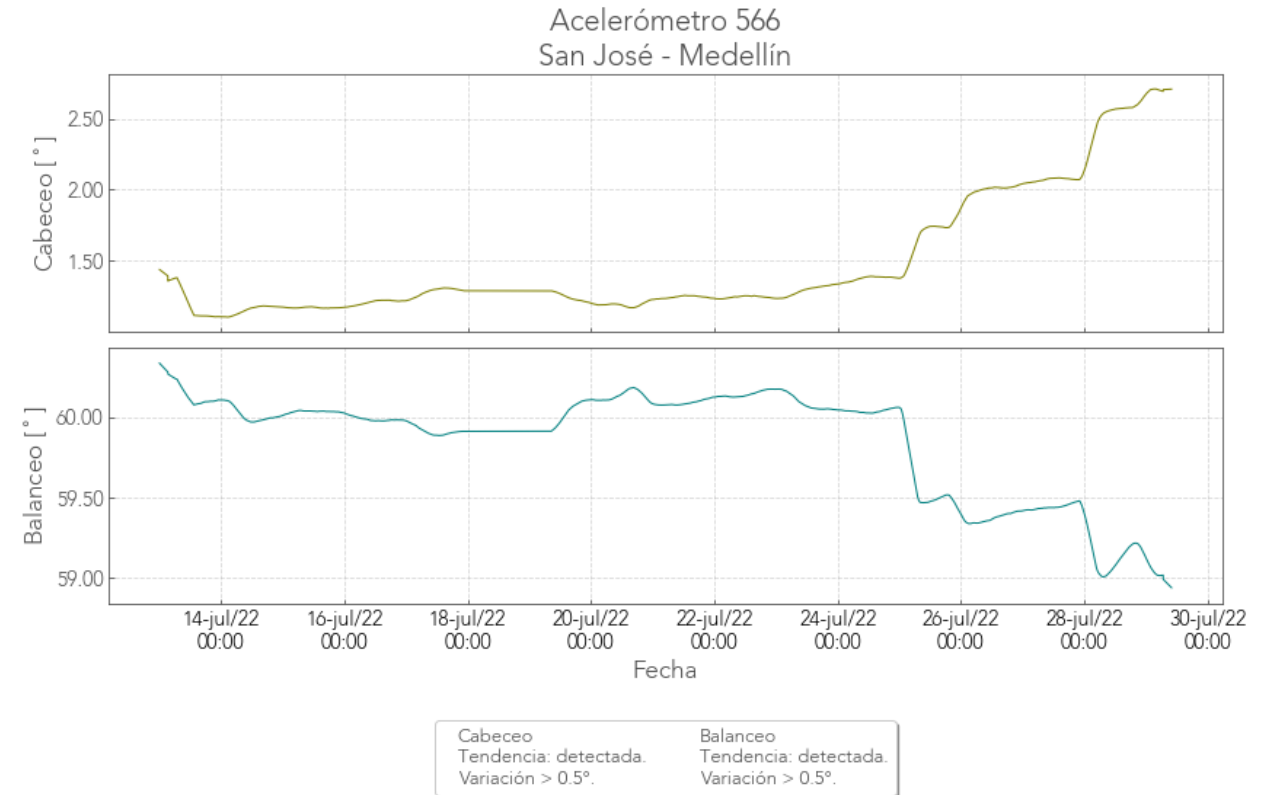
Figura 4. Registro del acelerómetro 566 San José-Medellín.
