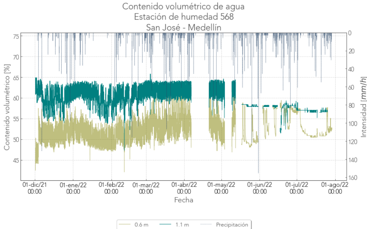
Figura 12. Registro histórico del sensor de humedad 568. Tanque vereda San José.
