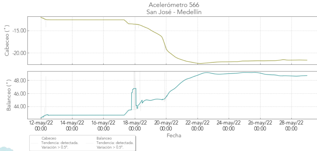
Figura 3. Registro del acelerómetro 566 San José-Medellín.
