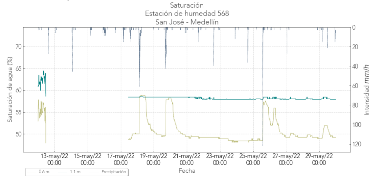
Figura 6. Registro sensor de humedad 568 San José-Medellín.
