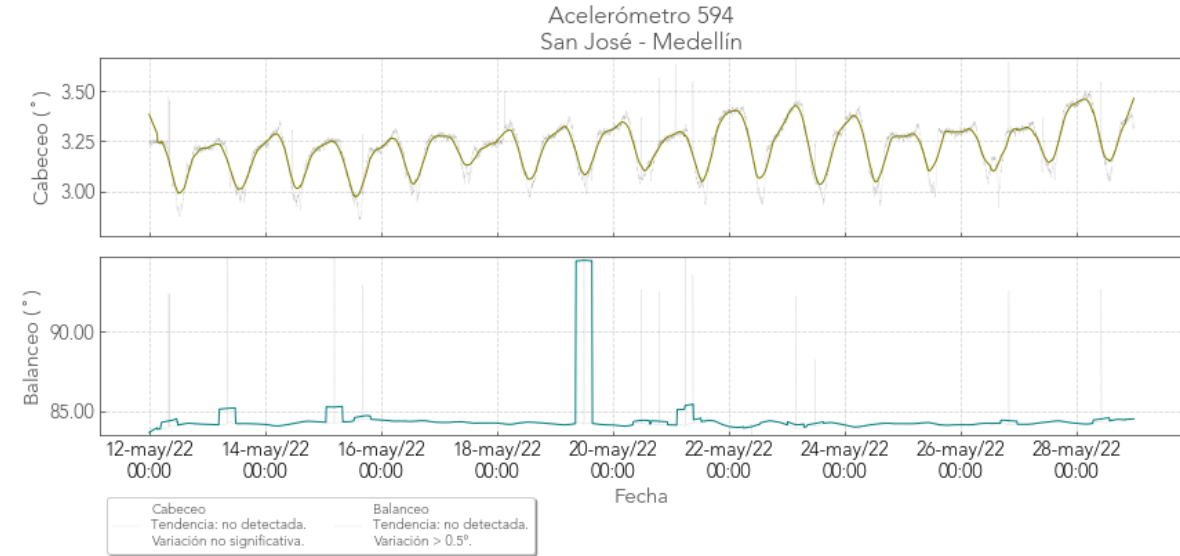
Figura 4. Registro acelerómetro 594 San José-Medellín.
