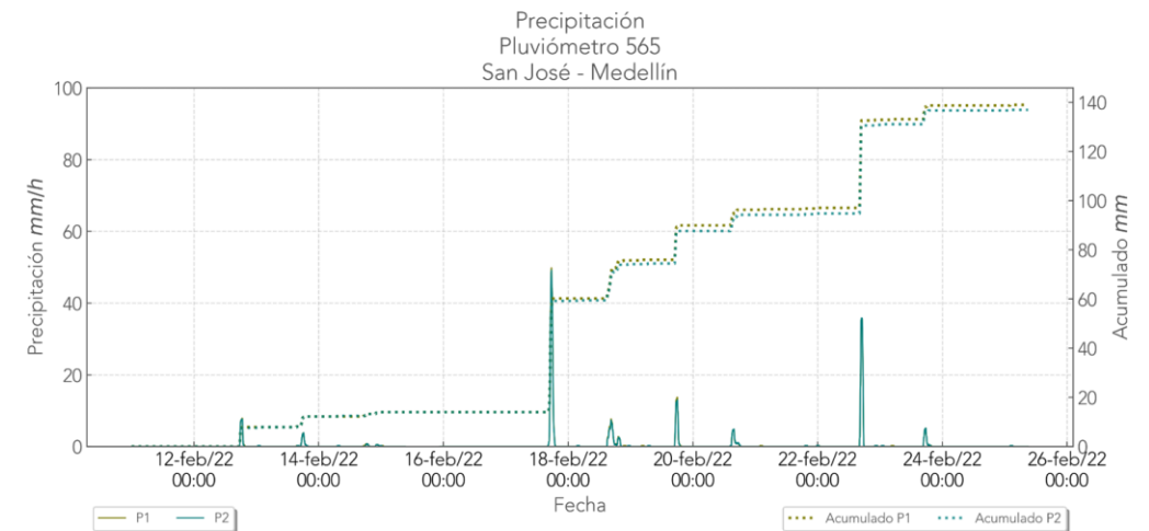
Figura 2. Registro pluviométrico entre el 11 y 25 de febrero de 2022 en el sector.
