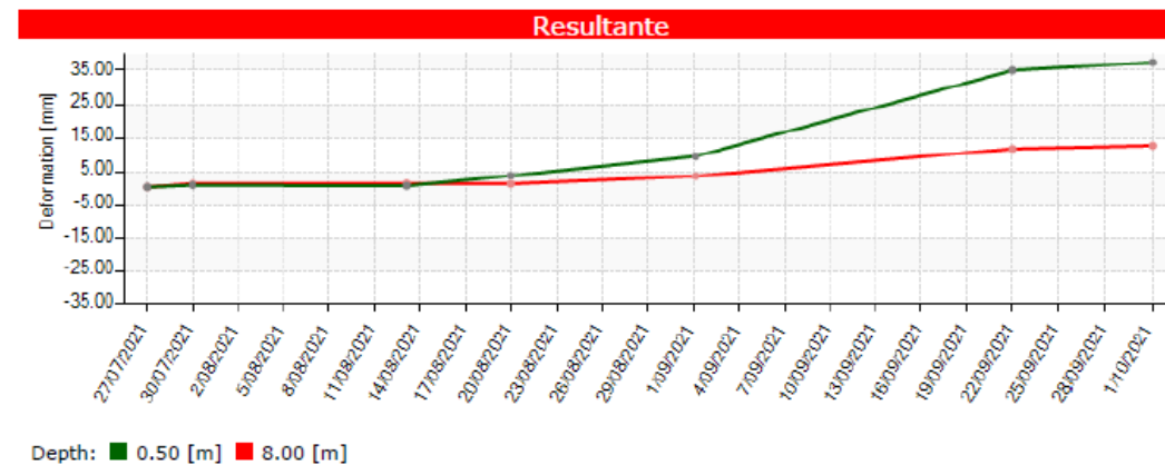
Figura 3. Evolución del desplazamiento del inclinómetro VP INC-02
