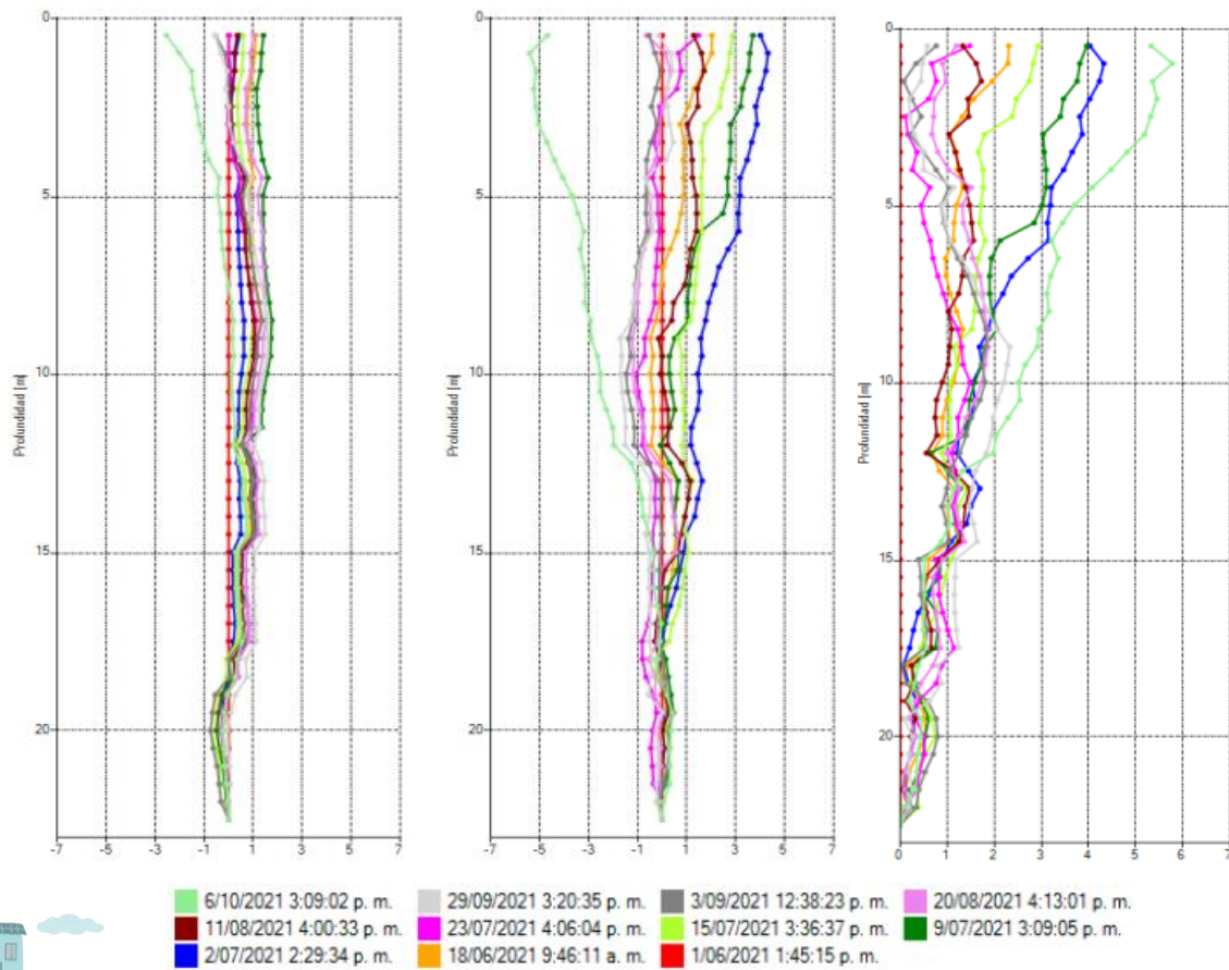
Figura 3. Desplazamientos relativos acumulados durante las mediciones realizadas.
