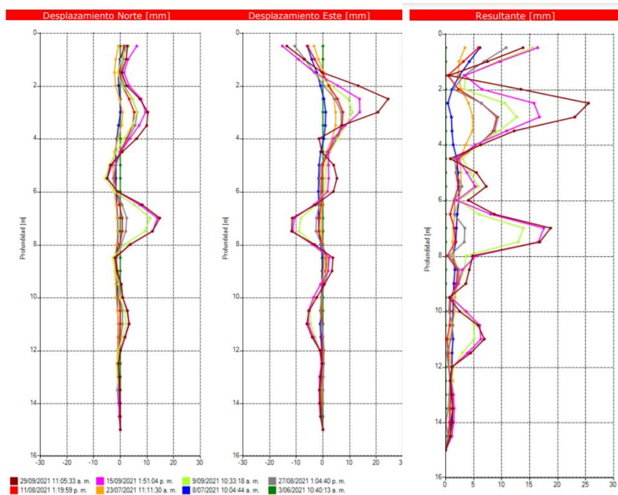
Figura 2. Desplazamientos relativos respecto al norte y al este. .
