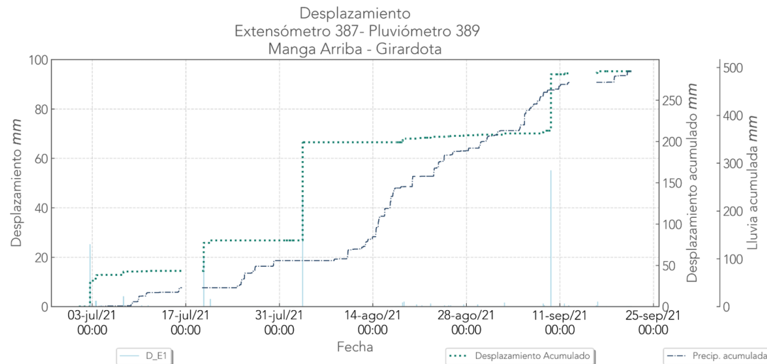
Figura 1. Desplazamiento superficial acumulado entre los meses de Julio a Septiembre en el extensómetro 387, ubicado en la finca El Tesoro.
