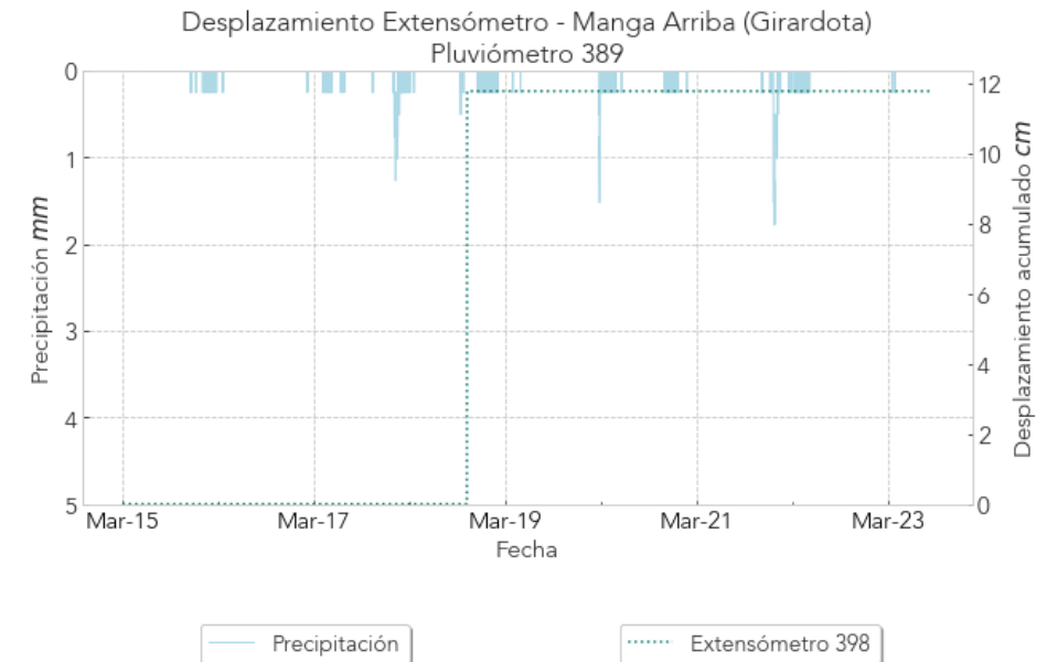
Figura 2. Desplazamiento superficial acumulado durante lo corrido de Marzo en el extensómetro 398.
