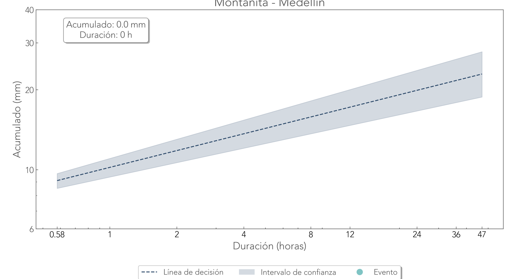
Comparación Acumulado-Duración Pluviómetro 519 Montanita - Medellín
