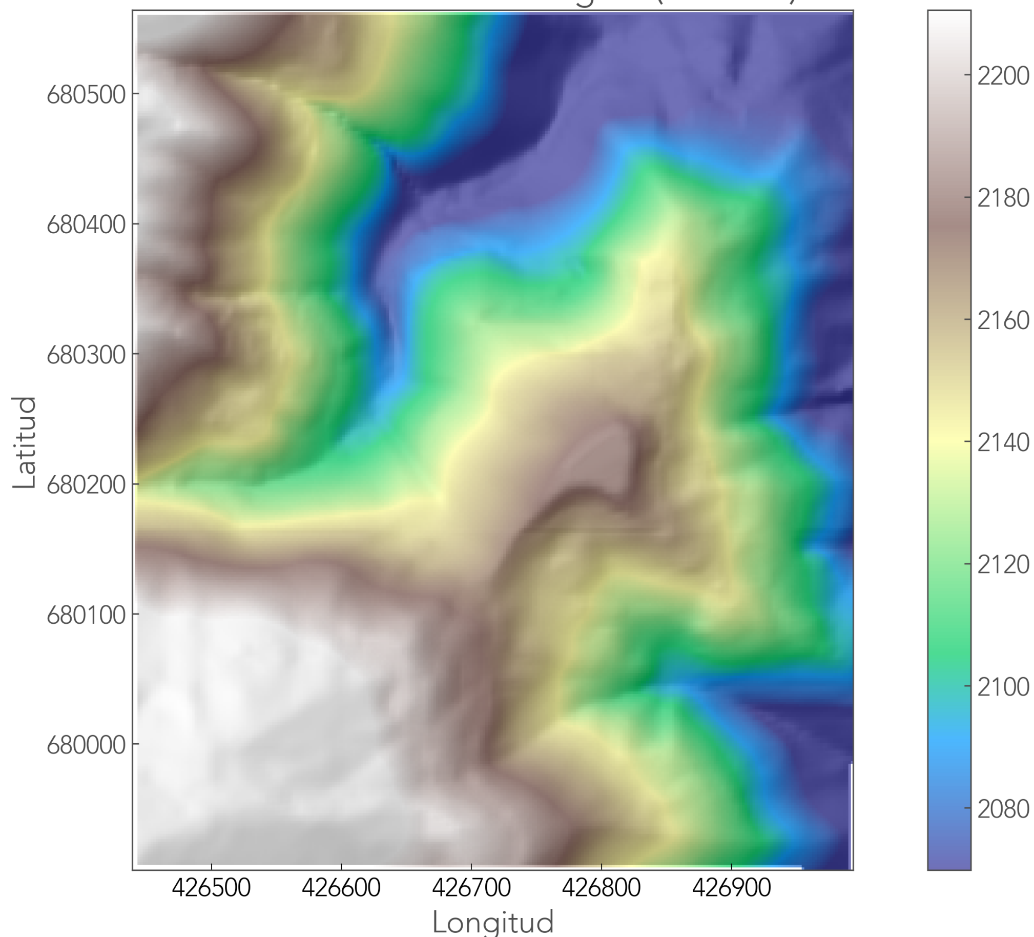
Modelo de Elevación Digital (m.s.n.m)
