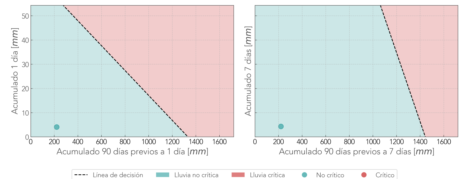
Comparación Reciente-Antecedente Pluviómetro 519 Montanita - Medellín
