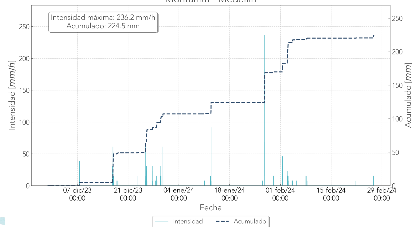
Precipitación Pluviómetro 519 Montanita - Medellín
