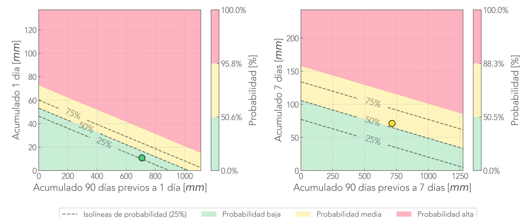
Comparación Reciente-Antecedente Pluviómetro La Lomita Parte Alta - Medellin
