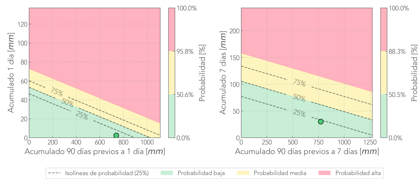
Comparación Reciente-Antecedente Pluviómetro Tierra Alta - Medellín
