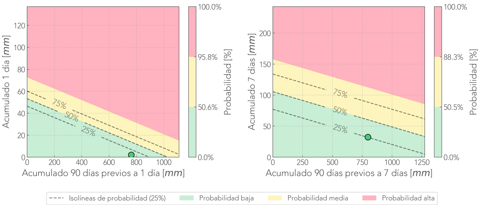
Comparación Reciente-Antecedente Pluviómetro La Montana - Medellín
