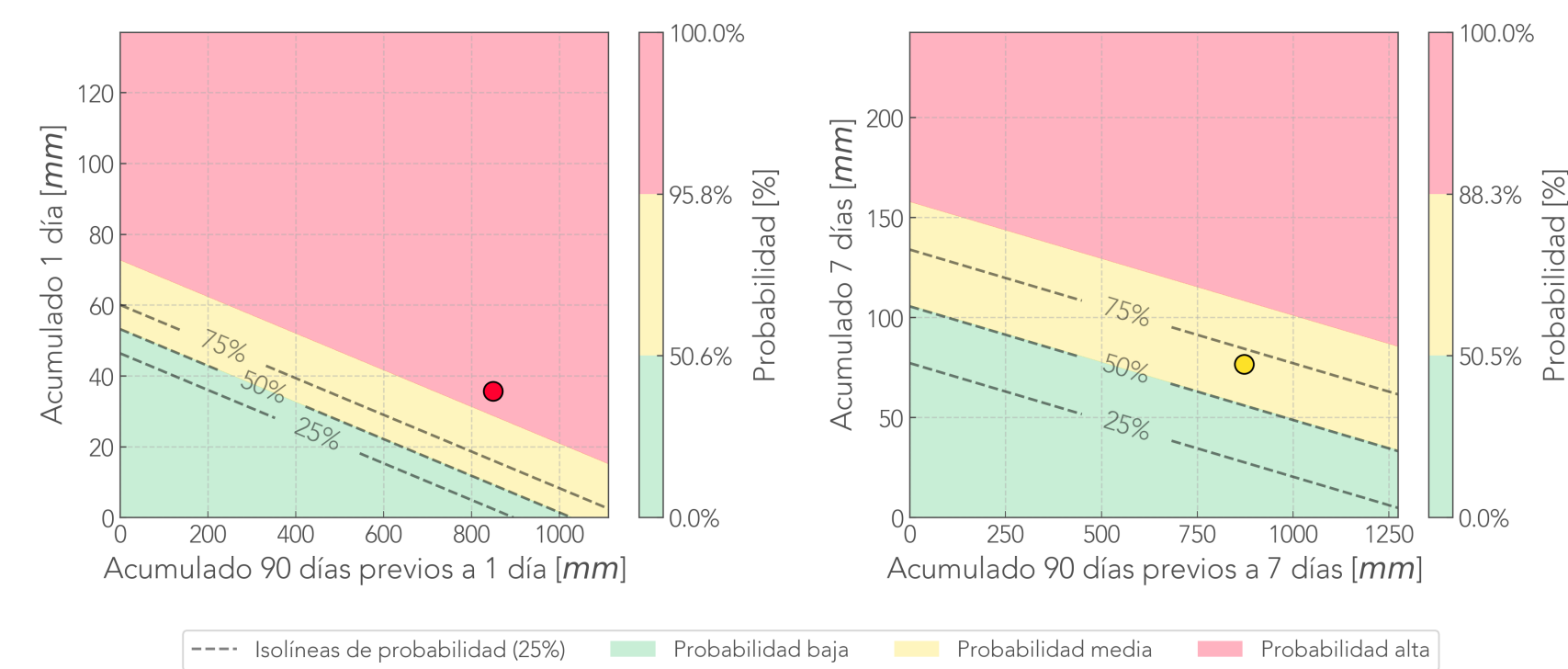
Comparación Reciente-Antecedente Pluviómetro La Fortuna Parte Alta - Medellín
