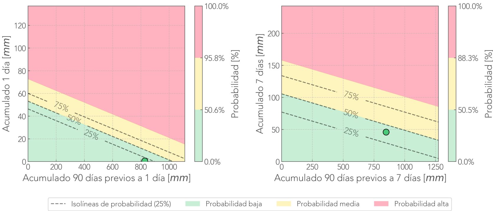
Comparación Reciente-Antecedente Pluviómetro Parqueadero Barichara - Medellín
