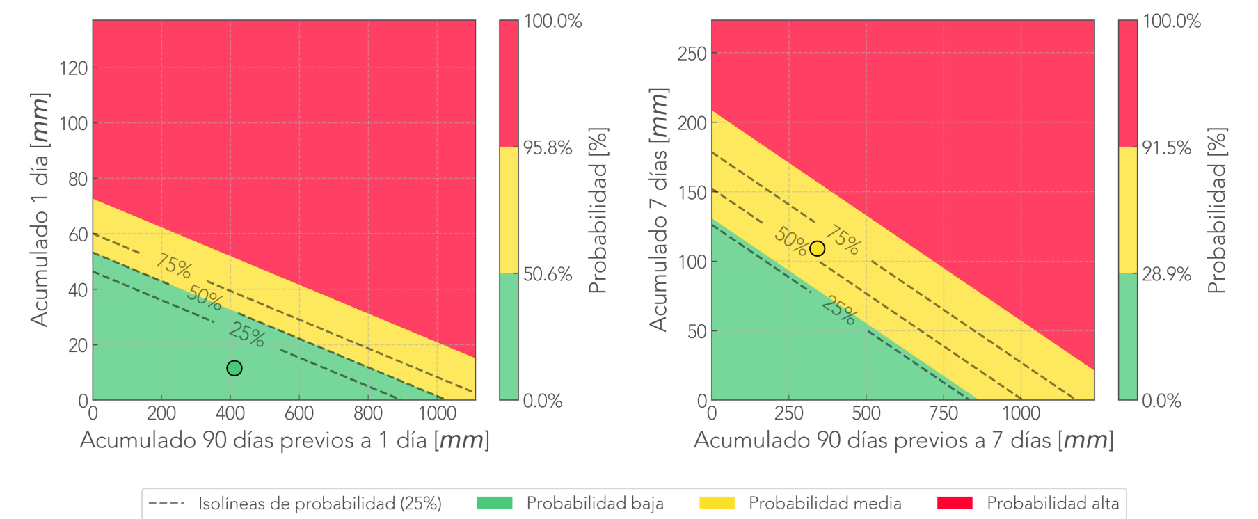
Comparación Reciente-Antecedente Pluviómetro El Hatillo - Barbosa
