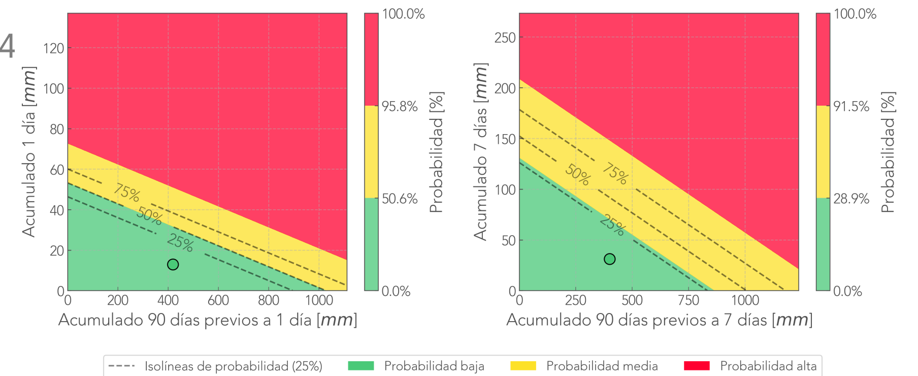
Comparación Reciente-Antecedente Pluviómetro La Sanin - Medellín
