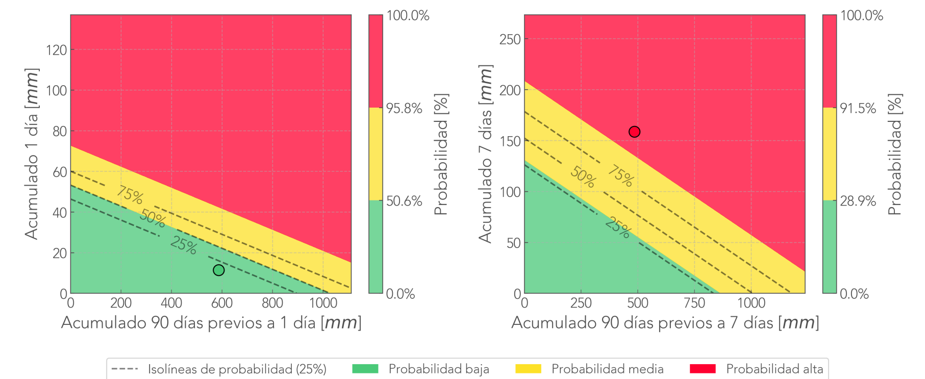
Comparación Reciente-Antecedente Pluviómetro ElSalado - Medellín
