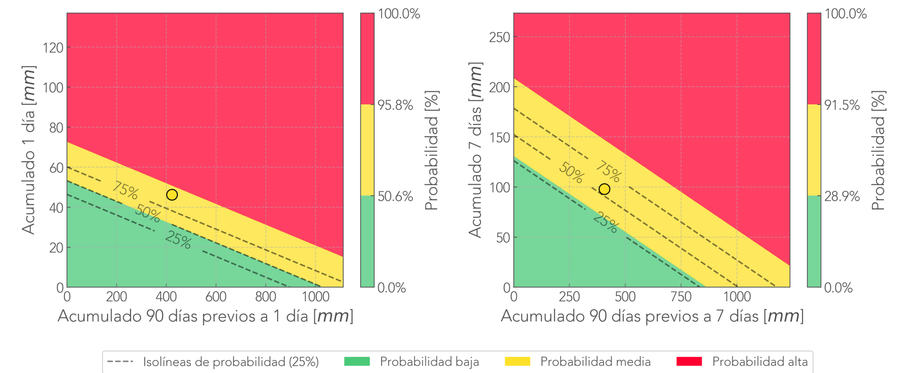
Comparación Reciente-Antecedente Pluviómetro El Pacífico - Medellín
