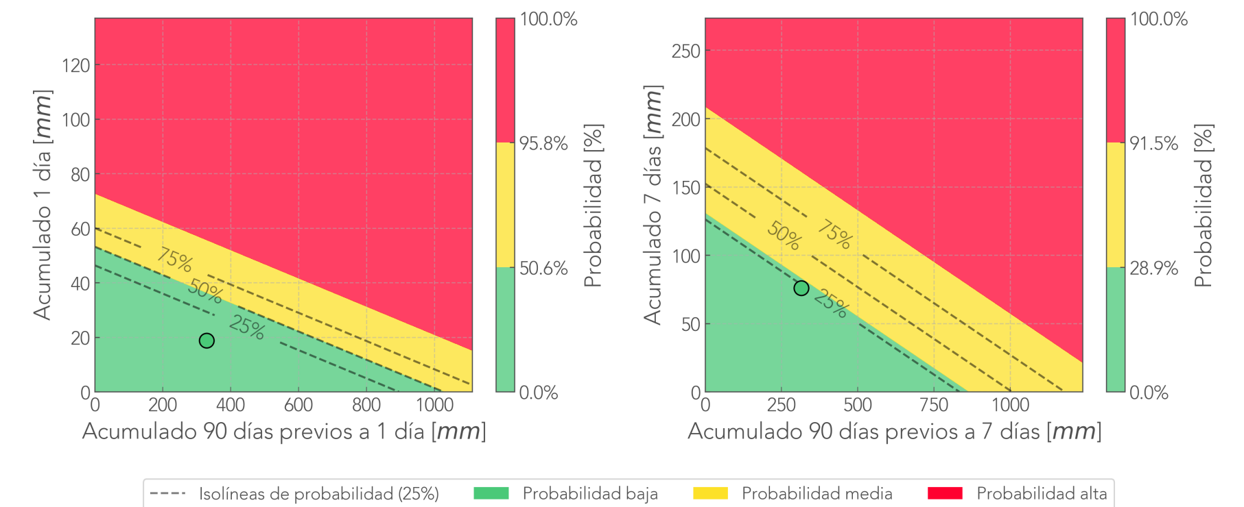
Comparación Reciente-Antecedente Pluviómetro Emergencia Metro - Medellín
