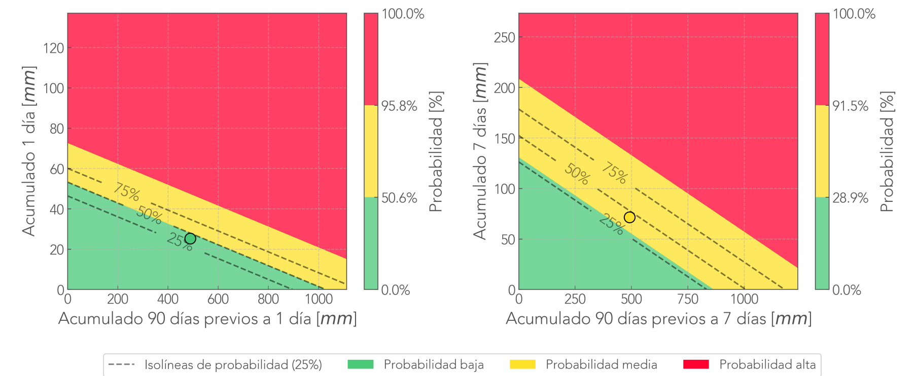
Comparación Reciente-Antecedente Pluviómetro AnimalX - Medellín
