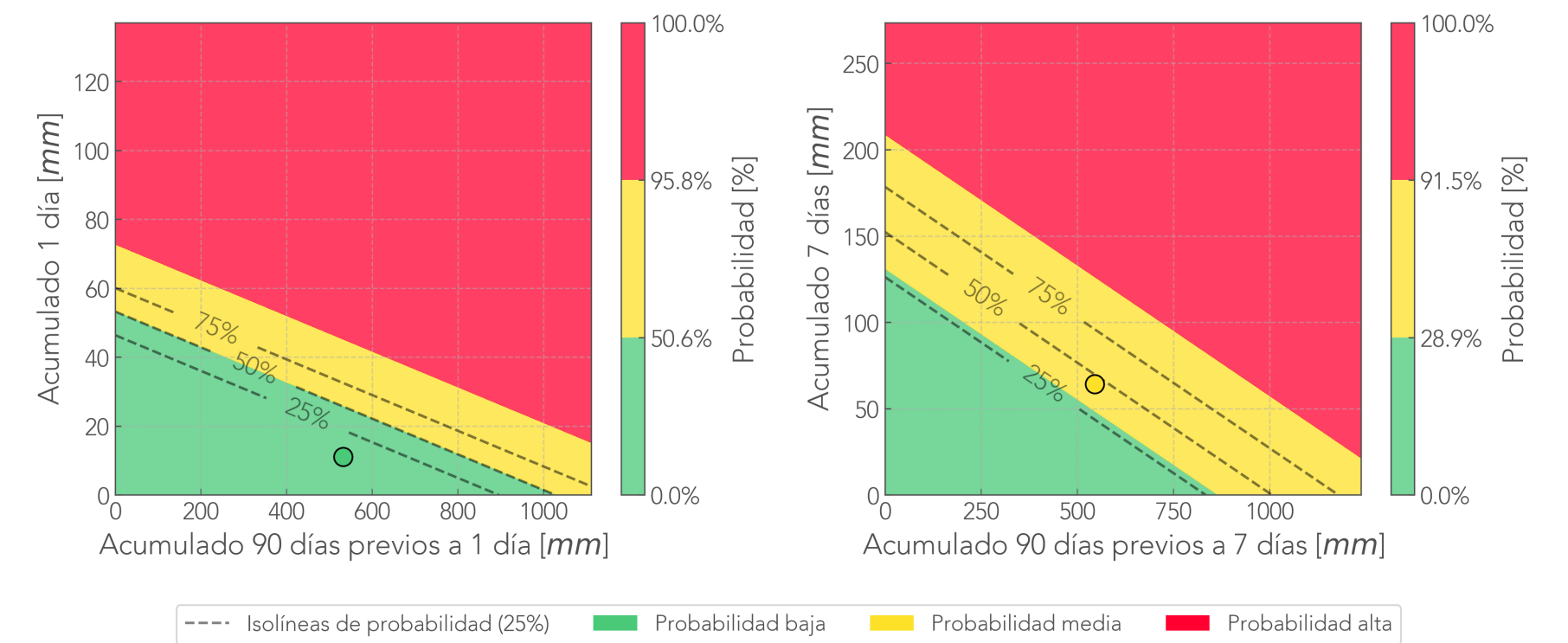
Comparación Reciente-Antecedente Pluviómetro Ajizal - Itagüí
