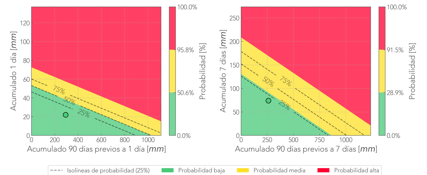
Comparación Reciente-Antecedente Pluviómetro Potrerito - Bello
