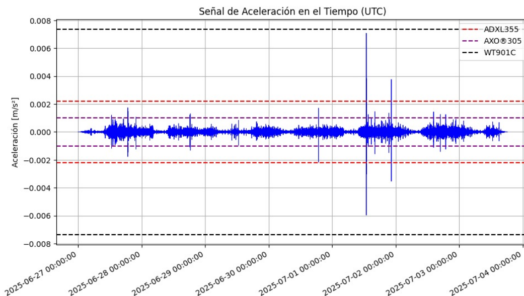
Figura 27. Comparación señal de geófono vs nivel de ruido de sensores
