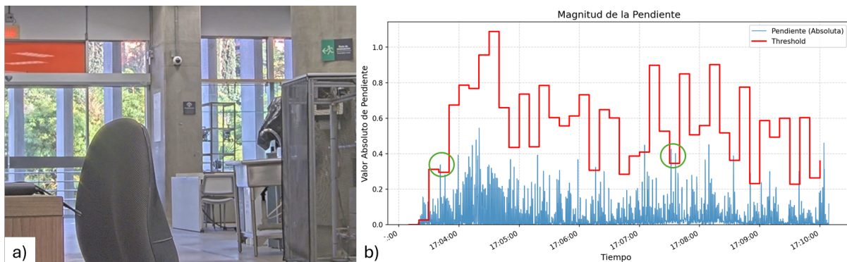
Figura 41. Análisis en entorno controlado a) Campo de visión, b) Magnitud de la pendiente y umbral adaptativo sin mínimo
