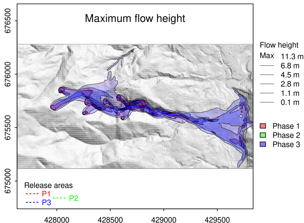
Figura 18. Modelación basada en zonas fuentes y sus parámetros geotécnicos del tránsito con avaflow para la cuenca La Raya.
