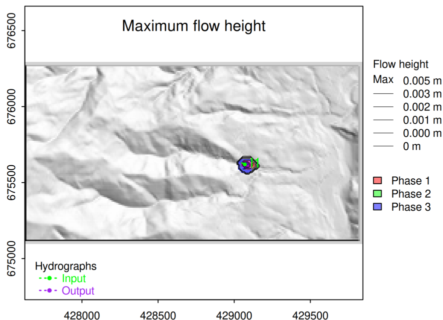
Figura 19. Modelación basada en hidrograma para un período de retorno de 5 años del tránsito con avaflow para la cuenca La Raya.
