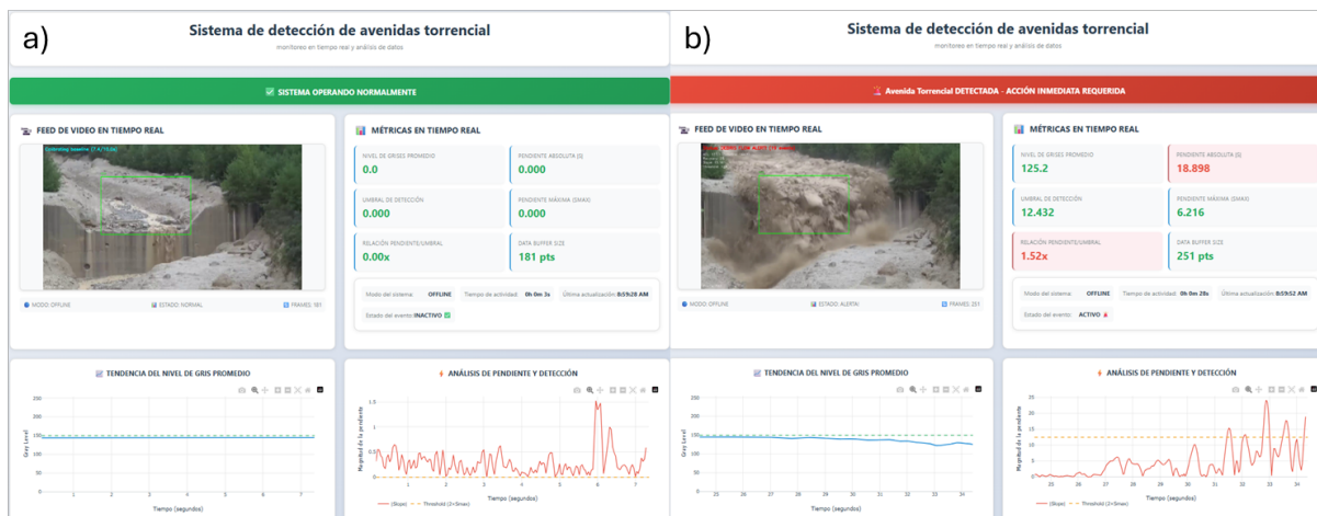
Figura 40. Interfaz procesamiento de imágenes en modo offline a) el frente de la avenida torrencial no ha sido captado por la cámara, b) el frente de la avenida torrencial llega a la visual de la cámara
