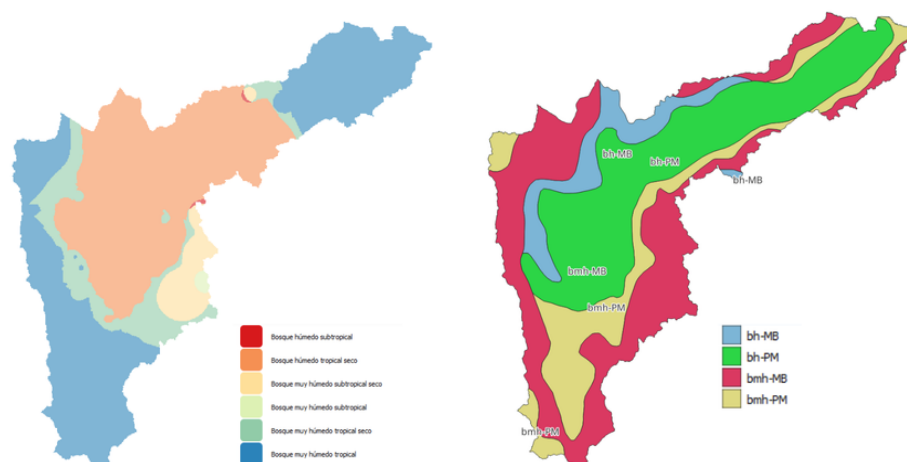
Figura 3.2. Comparación entre las zonas de vida obtenidas con la primera aproximación (izquierda) y las zonas de vida oficiales del IGAC (derecha). Se observan inconsistencias asociadas al campo de ETP.
