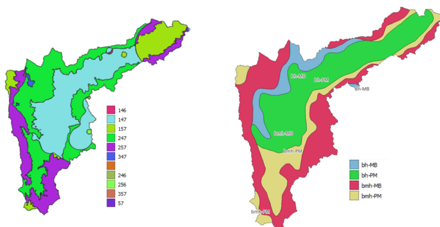
Figura 3.4. Comparación entre las zonas de vida obtenidas con el método alternativo (izquierda) y las zonas de vida oficiales del IGAC (derecha). Se observan inconsistencias.
