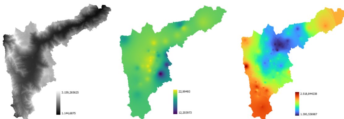
Figura 3.3. Mapas de altitud (DEM), temperatura y precipitación empleados en la clasificación de zonas de vida según la “Clasificación de suelos de Antioquia”.
