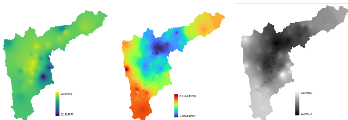
Figura 3.1. Mapas de temperatura media anual, precipitación anual y evapotranspiración potencial (ETP) empleados en la primera aproximación de zonas de vida.
