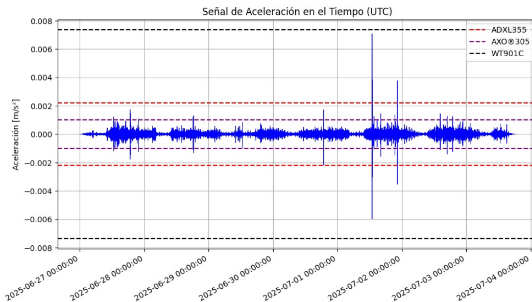
Figura 21. Comparación señal de geófono vs nivel de ruido de sensores
