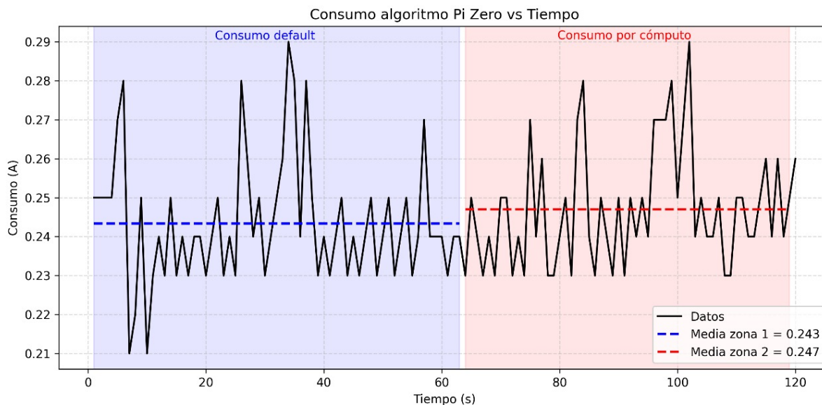
Figura 31. Consumo eléctrico en estado basal y bajo procesamiento de algoritmo de señales del geófono en una Raspberry Pi Zero
