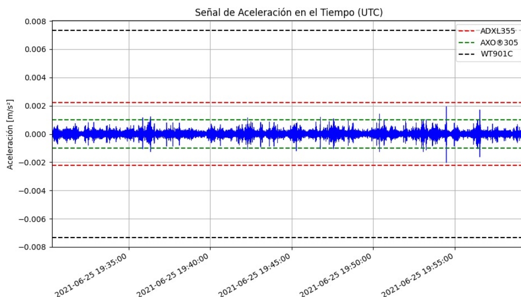
Figura 22. Señal de evento de avenida torrencial captada por un geófono [REF Sebas] y niveles rms de ruido de acelerómetros e IMU
