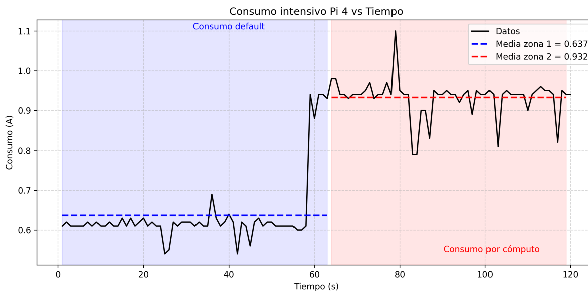
Figura 26. Consumo eléctrico en estado estático y bajo alta demanda computacional en una Raspberry Pi 4.
