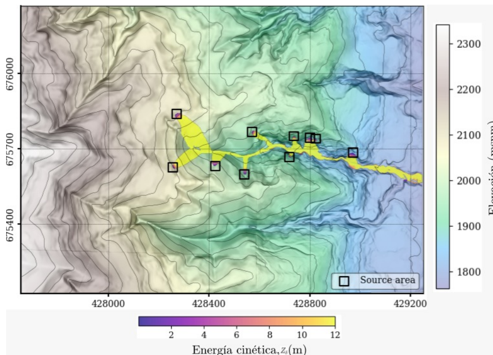
Figura 13. Modelación del tránsito con Flow-Py para la cuenca La Raya.
