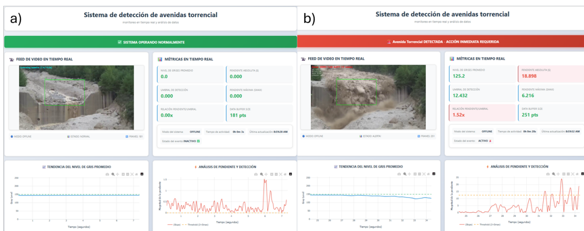
Figura 33. Interfaz procesamiento de imágenes en modo offline a) el frente de la avenida torrencial no ha sido captado por la cámara, b) el frente de la avenida torrencial llega a la visual de la cámara
