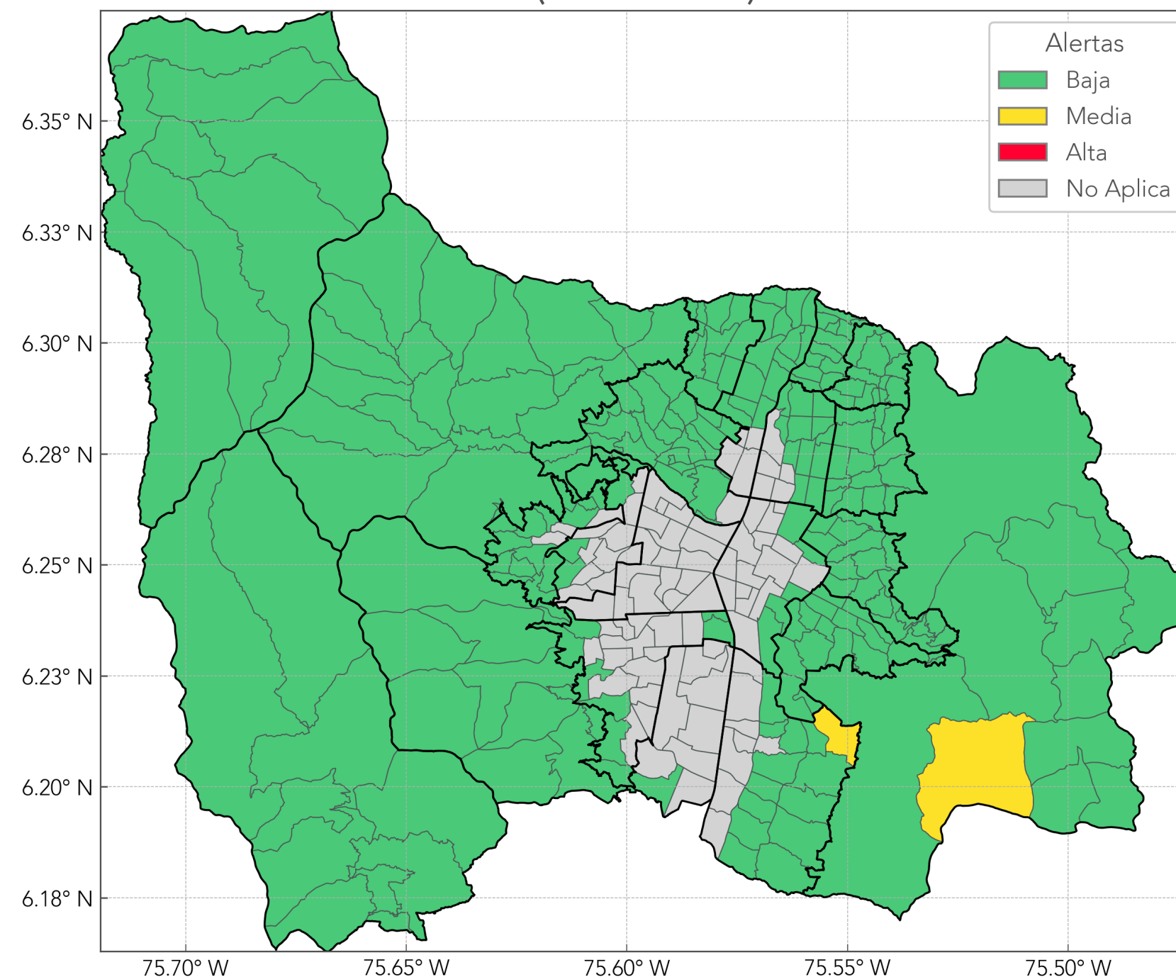
Probabilidad de ocurrencia de Movimientos en Masa (2026-02-09)
