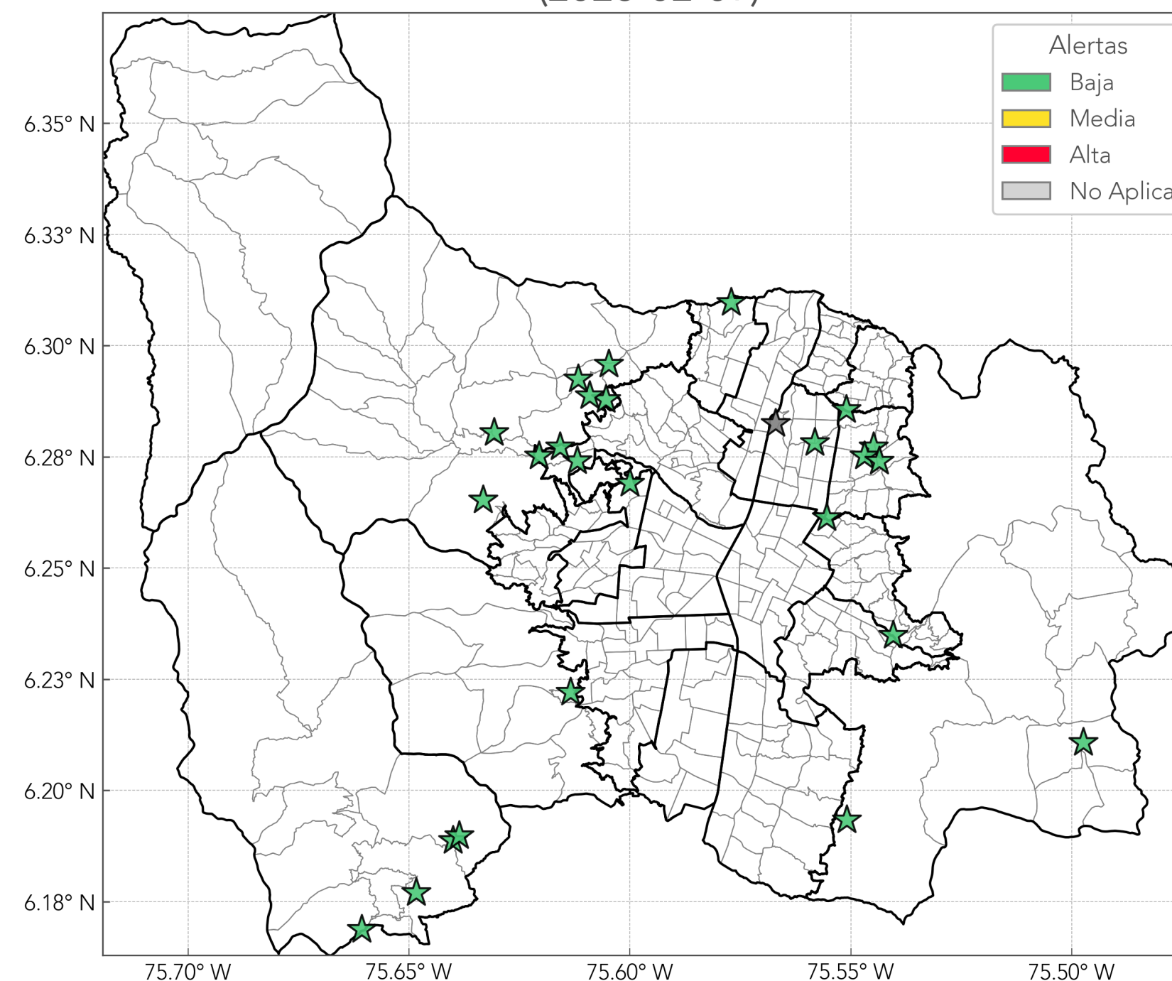
Probabilidad de ocurrencia de Movimientos en Masa (2026-02-09)
