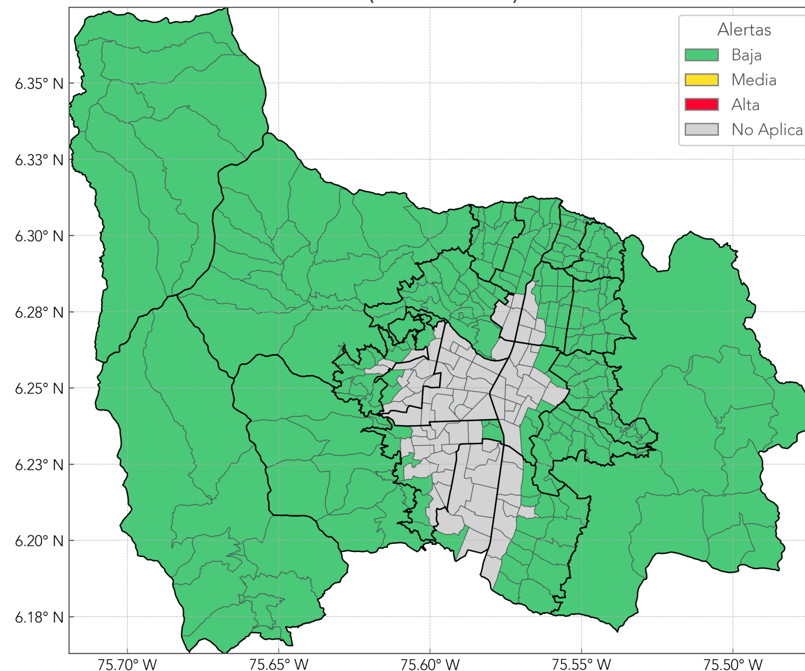
Probabilidad de ocurrencia de Movimientos en Masa (2025-12-26)
