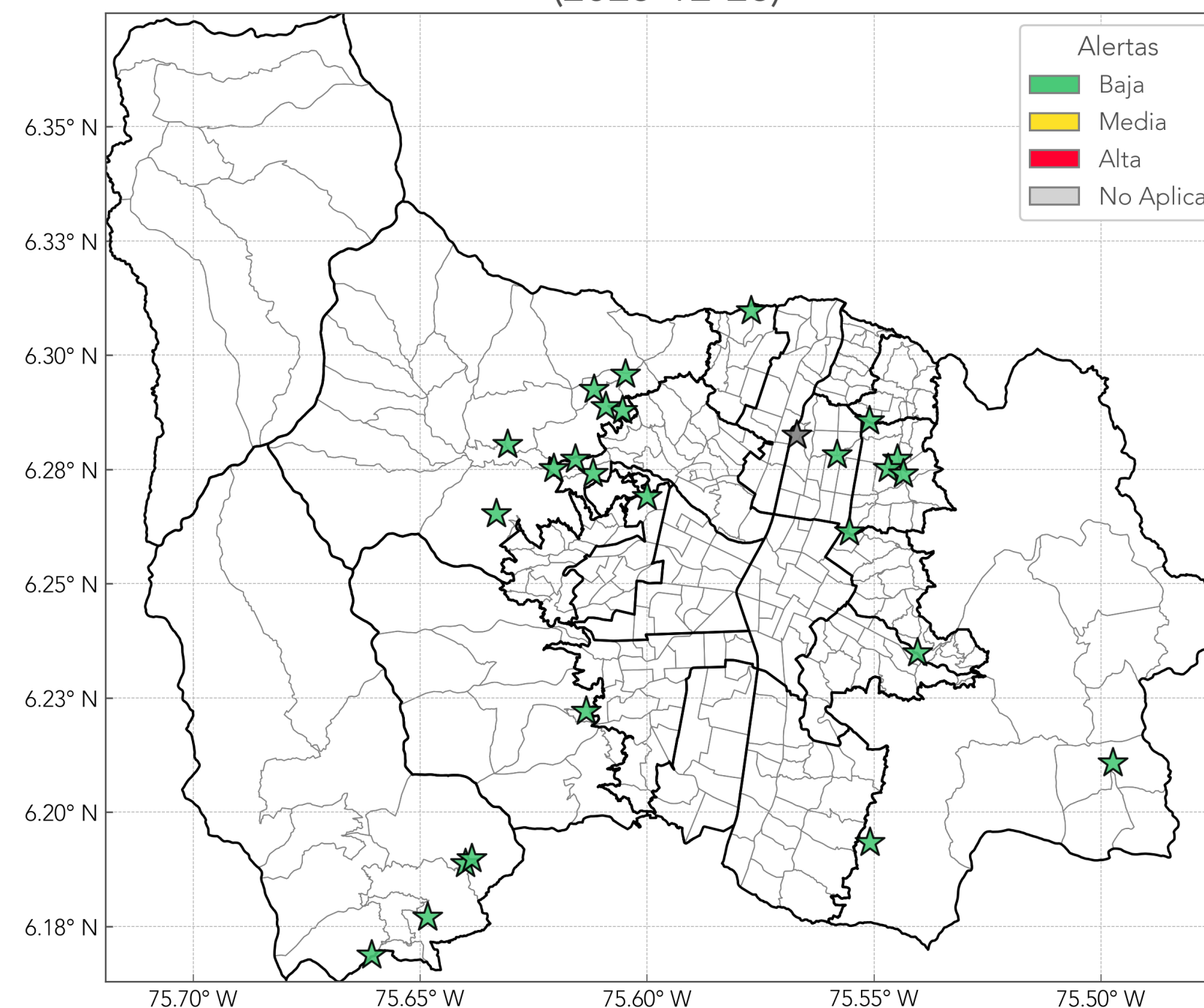
Probabilidad de ocurrencia de Movimientos en Masa (2025-12-26)
