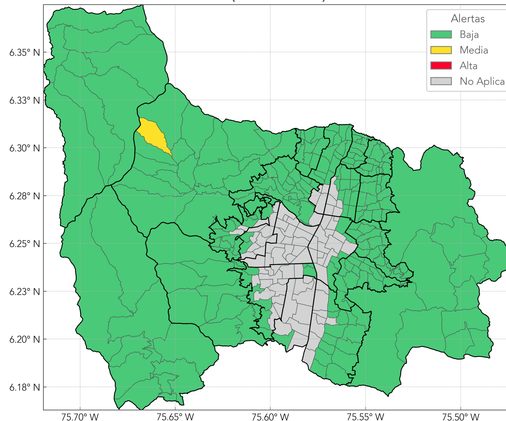
Probabilidad de ocurrencia de Movimientos en Masa (2025-12-01)
