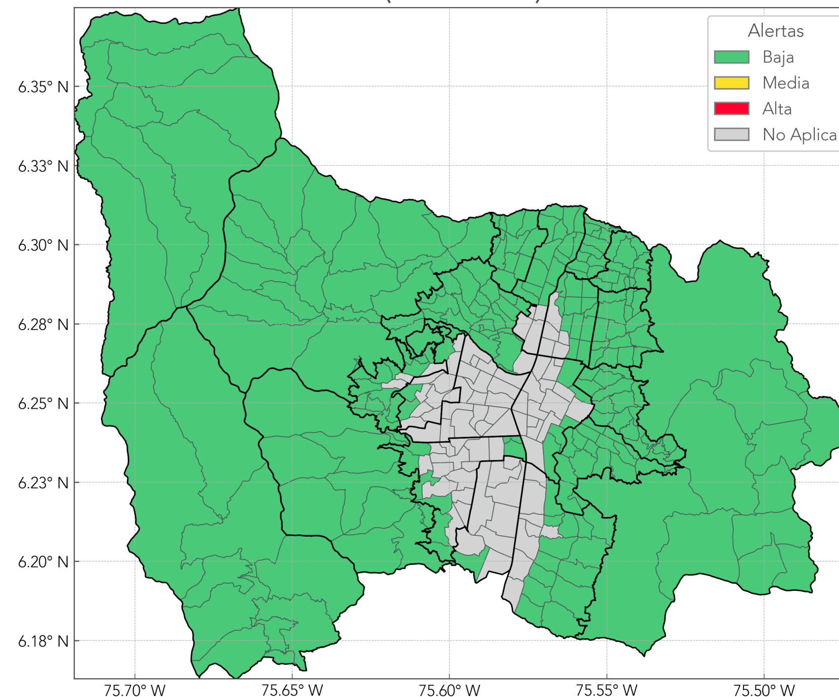
Probabilidad de ocurrencia de Movimientos en Masa (2025-10-20)
