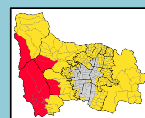
Mapa de alertas por movimientos en masa
