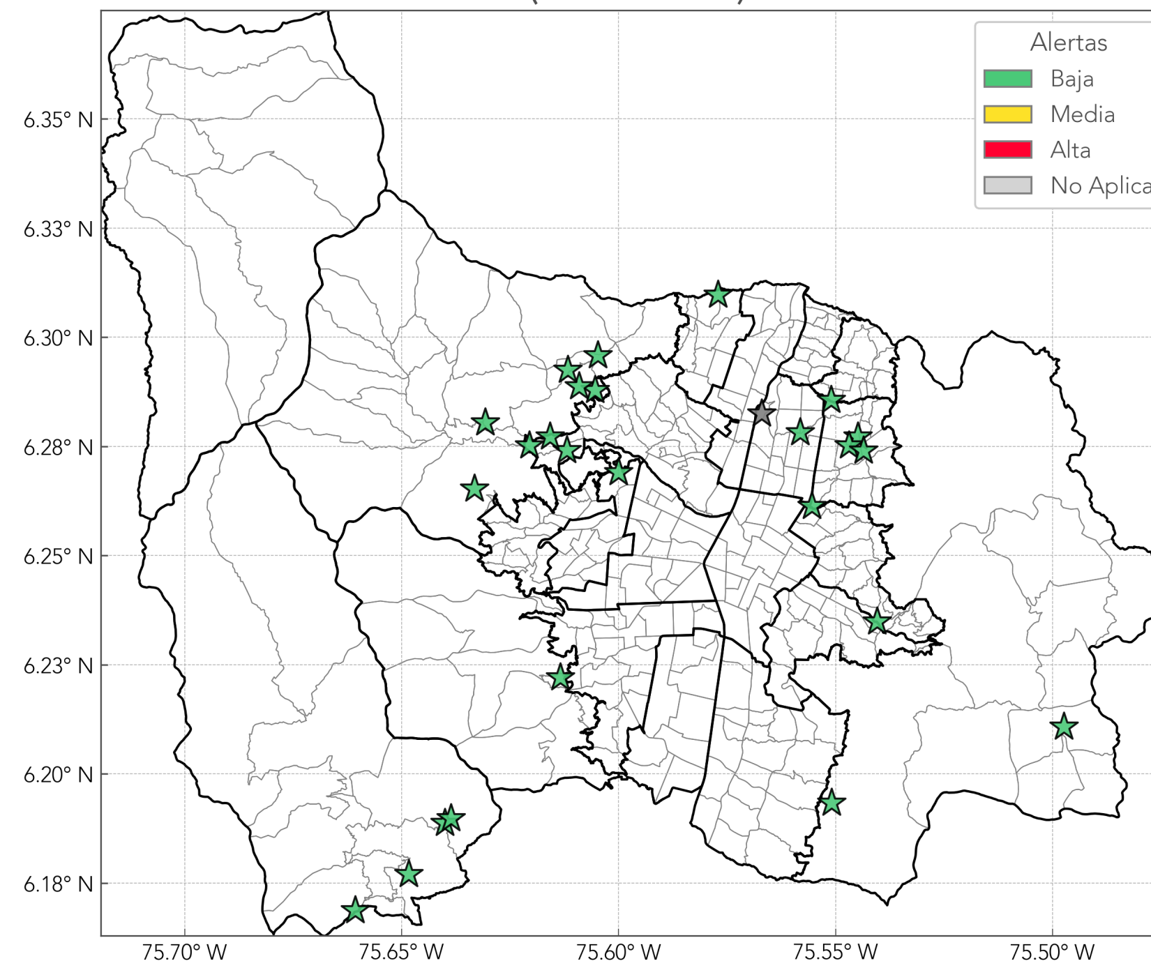
Probabilidad de ocurrencia de Movimientos en Masa (2025-10-13)
