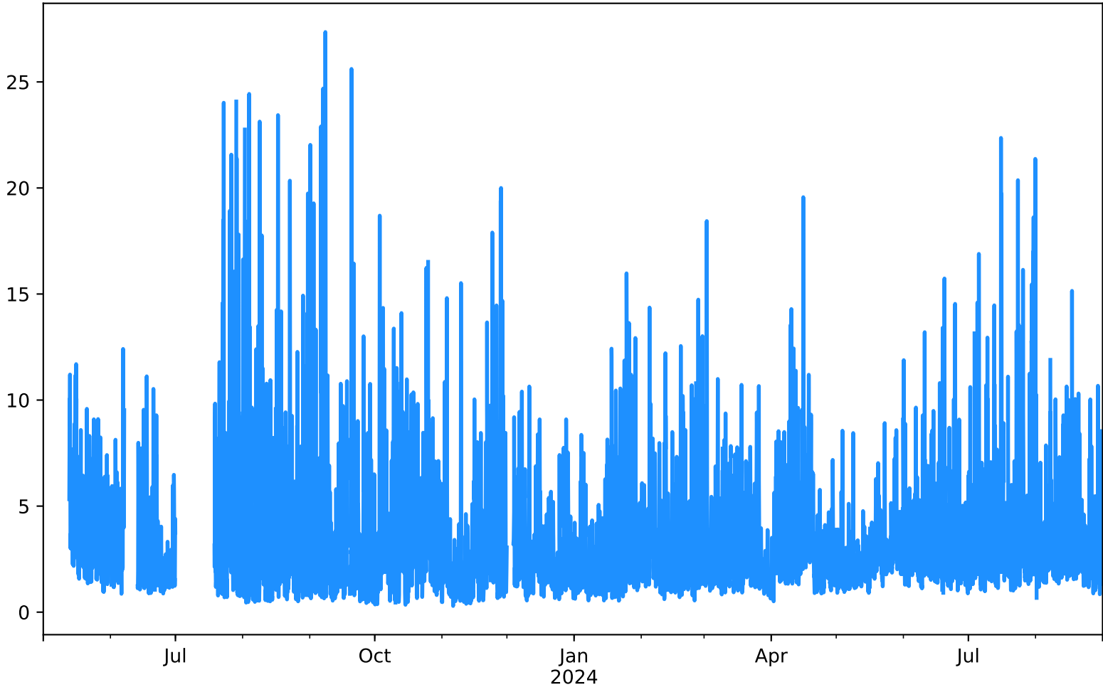
SO2 Estación ITA-CJUS Desde 2023-05-01 00:00 Hasta 2024-08-31 23:00
