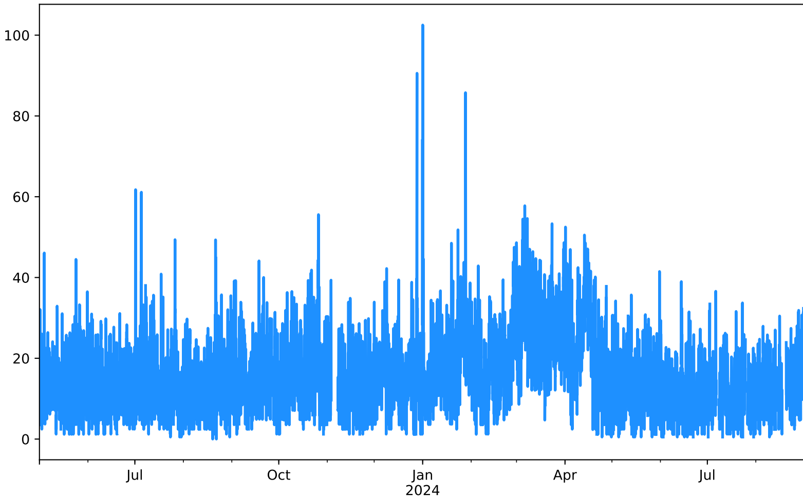
PM2.5 Estación BEL-FEVE Desde 2023-05-01 00:00 Hasta 2024-08-31 23:00
