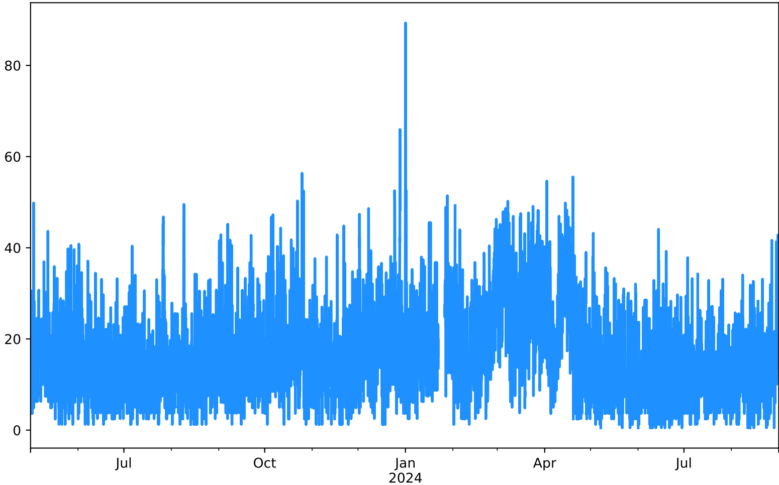
PM2.5 Estación MED-SCRI Desde 2023-05-01 00:00 Hasta 2024-08-31 23:00
